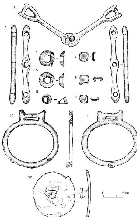
Рис. 2. Прорисовка бронзовых предметов конского снаряжения из кург. 31 Герасимовского могильника (художник Е. Печенегова).
