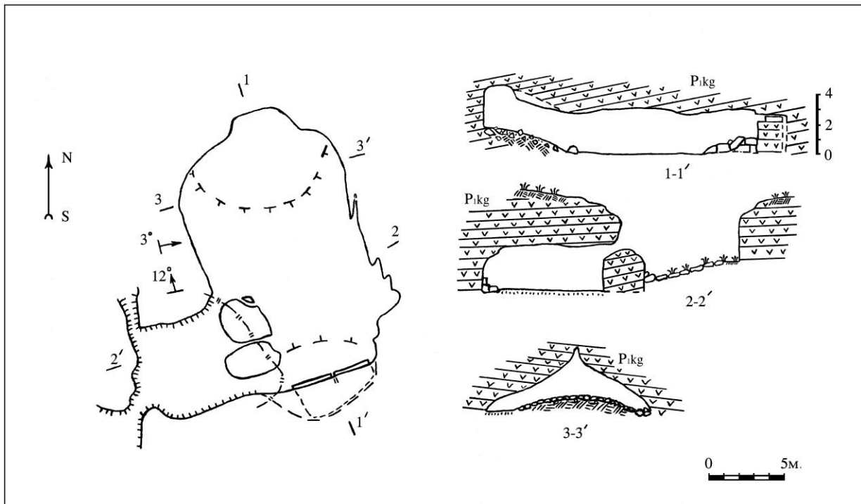
Рис. 2. План и разрезы пещеры Кененбай [2].
