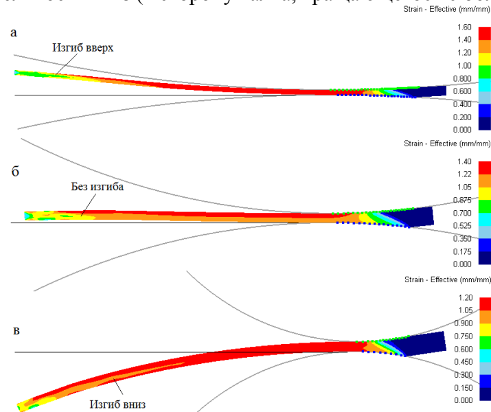
Рис. 3. Поле интенсивности деформации и направление изгиба полосы при различном параметре формы очага деформации: а) l_d/h_{cp} = 12,1 ; б) l_d/h_{cp} = 6,0 ; в) l_d/h_{cp} = 3,3
