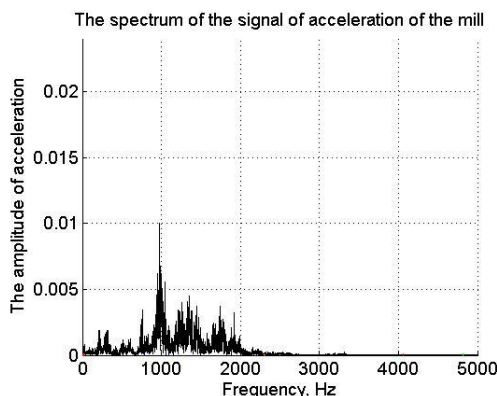
Рисунок 5 Фильтрованный спектр сигнала цапфы мельницы с загрузкой 400г
