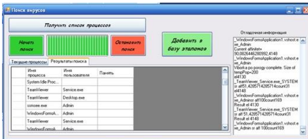
Рис 3. Алгоритм реализации
