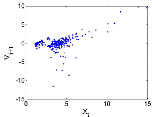
Рисунок 2 – Фазовый портрет «скорость – расстояние» при R_1 = 1 ; R_2 = 3 ; \gamma = 0,194 ; x_1 = 0,5
