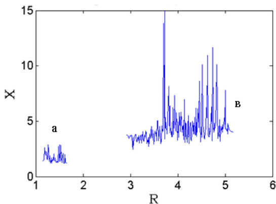
Рисунок 1 – Изменение размера галактик в зависимости от расстояния R а: формула (4), R_1 = 1 ; в: формула (5), R_2 = 3 .
