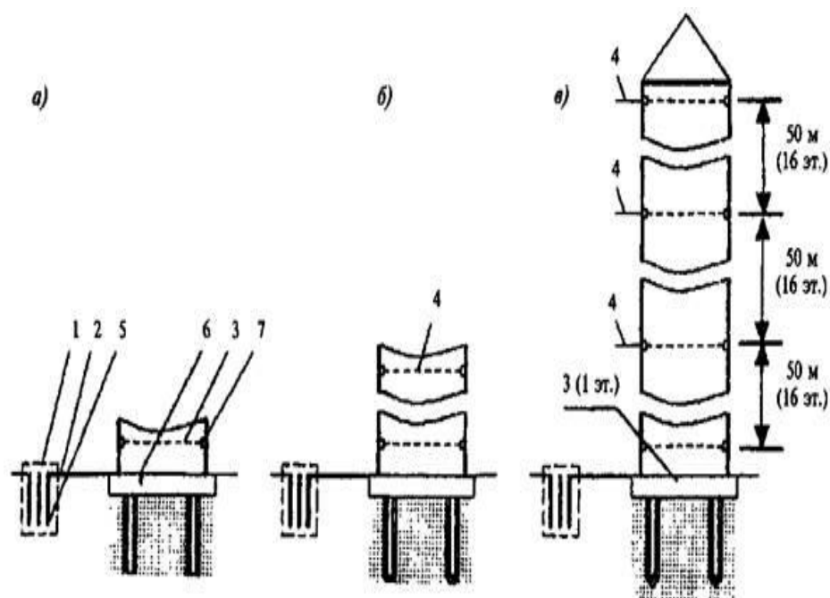
4 Сурет – Биік объектілерінің мониторингіннің типтік сұлбасы а-іргетасты орнату барысы; б-құрылысты орналастыру барысы; в-құрылыстың салынған кезі; 1-бастапқы биіктік кезеңі; 2-байлау кезеңі; 3-деформациялық тор; 4-монтаждық горизонттағы тор; 5-тереңдік репері; 6-едендегі отырған марка; 7-отырған марка; [4].
