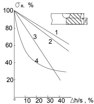
Рис. 1. Влияние относительной глубины \Delta h/s непровара корня шва на статическую прочность стыковых соединений (без выпуклости): 1 — Ст3; 2 — сталь 12X 18N9T; 3 — сталь 25XГФА; 4 — сплав Д16Т;
