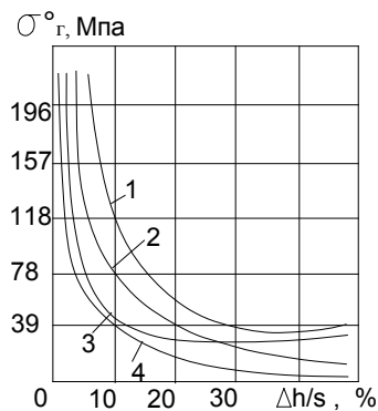
Рис. 2. Влияние относительной величины \Delta h/s дефектов на усталостную прочность стыковых соединений из низкоуглеродистых сталей (без выпуклости): 1 — подрезы; 2 — поры; 3 — непровар; 4 — шлаки. Где \Delta h — глубина непровара; s — толщина сварного шва.
