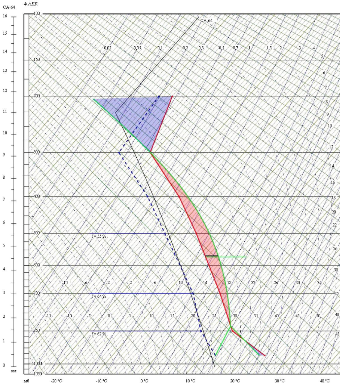
Рис. 1. Аэрологическая диаграмма, построенная при помощи программы ЗОНД
