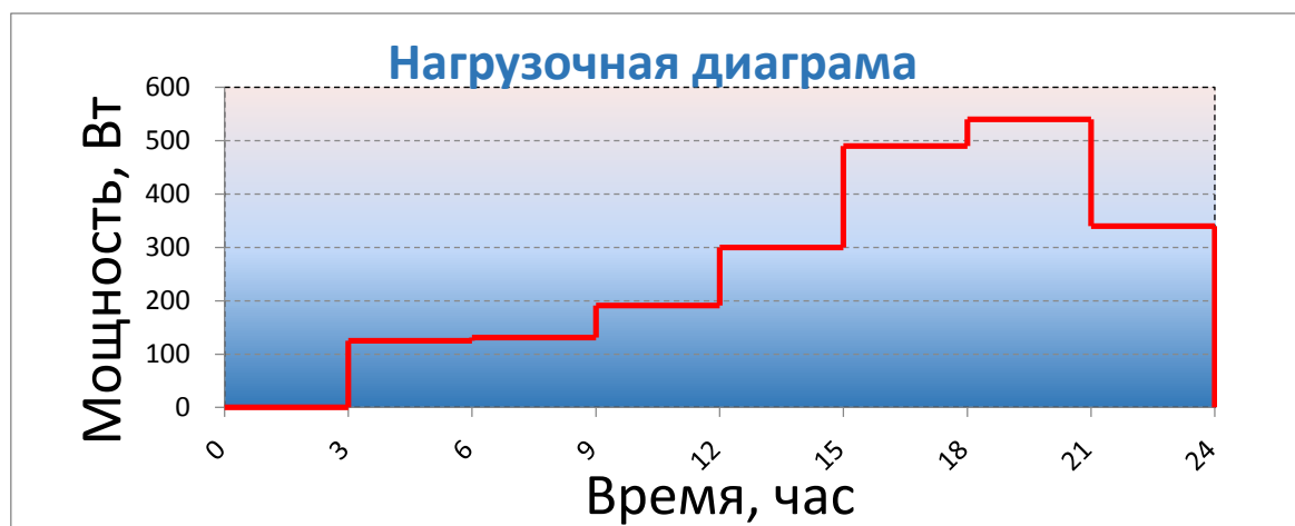
Рисунок 1 – Нагрузочная диаграмма суточного электропотребления
