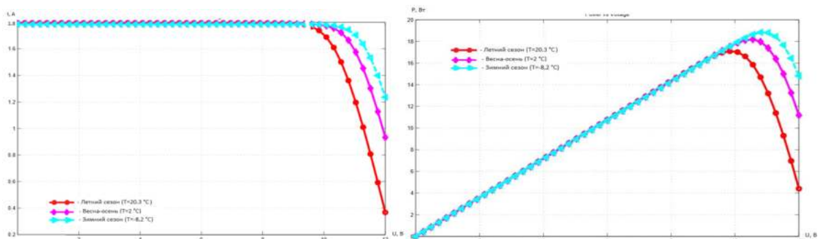
Рисунок 3 – Вольт-амперная и PV характеристики панели в зависимости от температуры воздуха по сезонам
