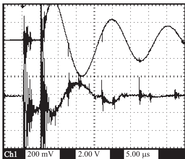
Рис. 3. Осциллограммы тока (112 кА/дел) и напряжения (20 кВ/дел) при давлении 0.1 Torr.
