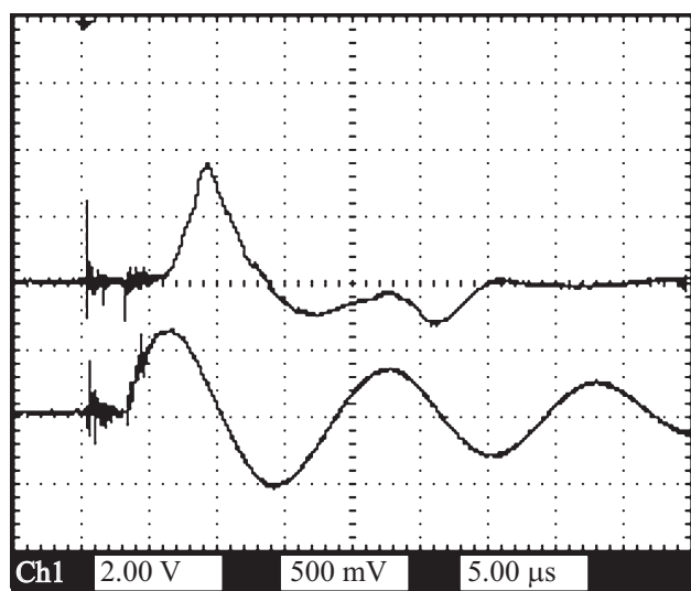
Рис. 6. Осциллограммы магнитного поля и разрядного тока (внизу).
