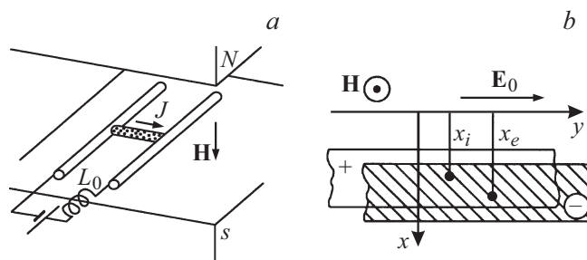
Рис. 2. Схемы рельсотрона (а) и двухблочной модели плазменного ускорителя по А.И. Морозову (b).
