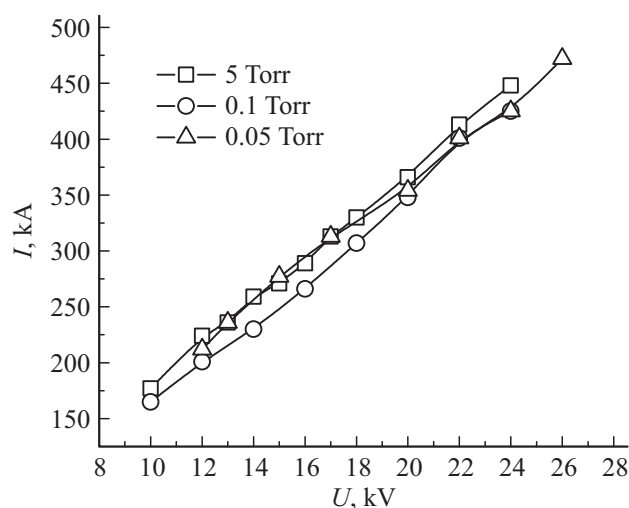
Рис. 4. Зависимость амплитуды разрядного тока от напряжения при различном давлении в камере ускорителя.
