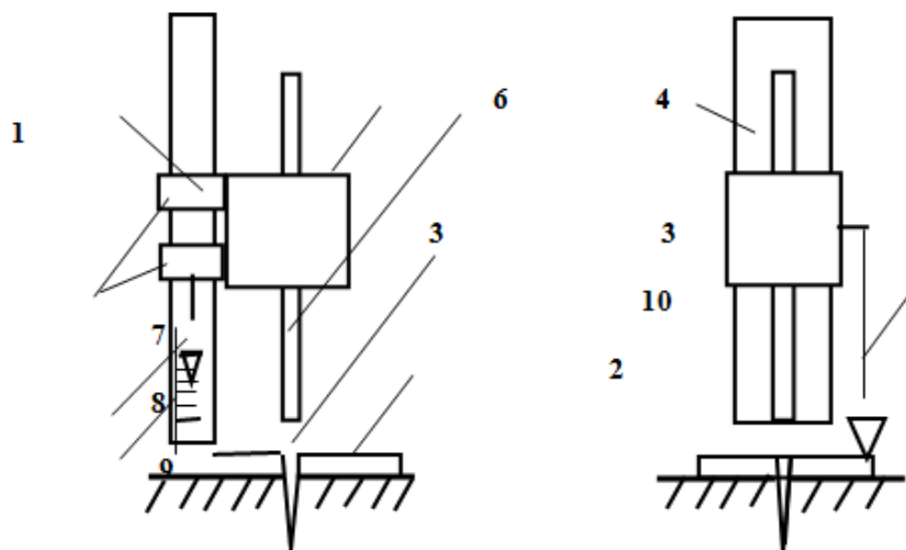
Рис.1 Схема макета «Плотномер».
