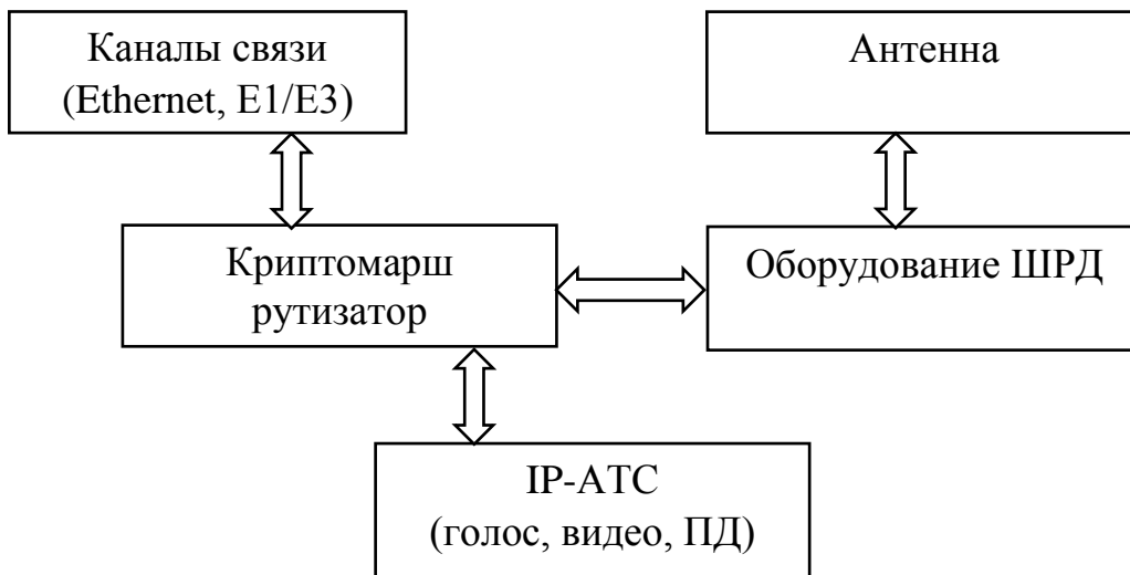
Рисунок 2- Вариант структуры элемента сети ШРД в комплексной аппаратной связи
