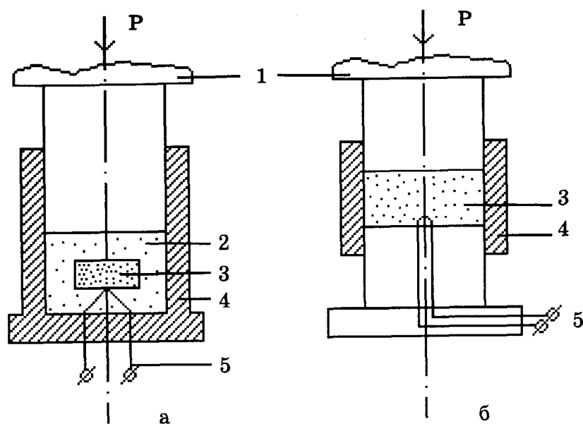
Рис. 38. Принципиальные схемы проведения процесса СВС-прессования: а — для тонких заготовок ; б — для крупногабаритных заготовок. 1—пуансон; 2—теплоизолятор; 3—шихта СВС; 4—пресс-форма; 5—инициирующее устройство.
