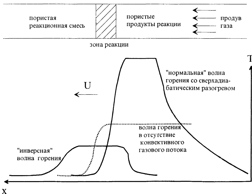
Рис. 14. Нормальная и инверсная волны горения при продуве газа через пористую среду
