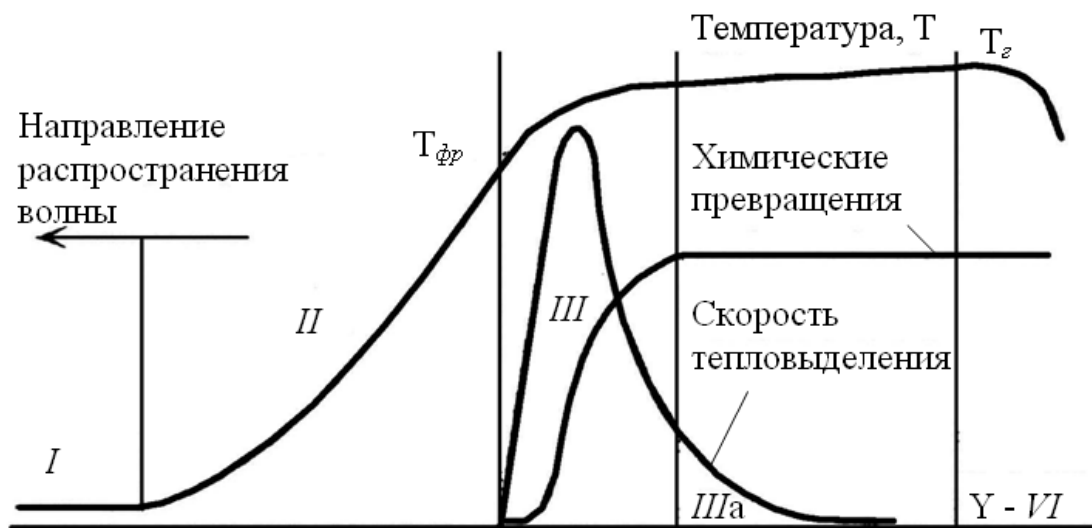
Рис. 3 Волновой комплекс в СВС – системе
