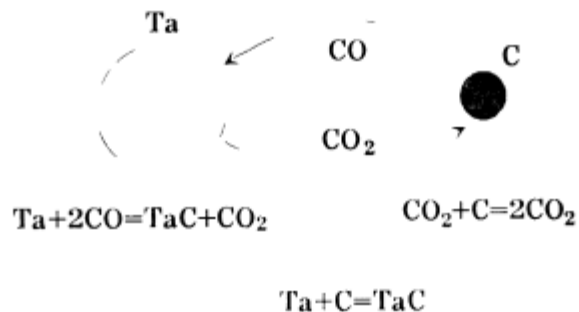
Рис. 11 Схема газофазного механизма в системе тантал-углерод
