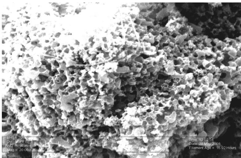
Рис.57- Частицы синтезированного кремния
