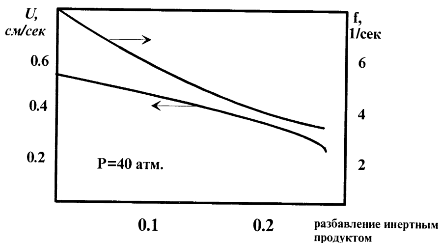
Рис. 10. Зависимость скорости горения системы Ta+xC от соотношения реагентов (x), давления газа (P), диаметра образца (D), содержания крупного тантала в смеси и разбавления (В.М. Шкиро и др.)
