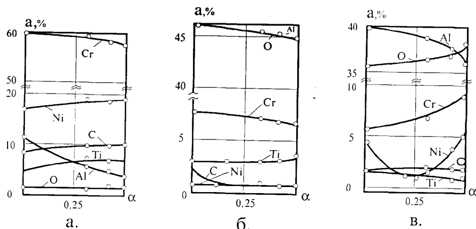
Рис. 45. Влияние состава исходной смеси а на химический состав металлической (а) шлаковой (б) и дисперсной (в) фаз. Исходная смесь: (1 - \alpha) (\text{CrO}_3 + \text{TiO}_2 + \text{NiO} + \text{Al} + \text{C}) + \text{Cr}_2\text{O}_3
