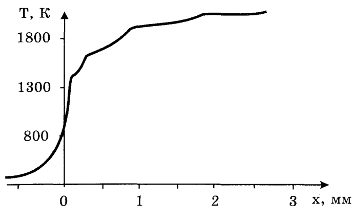
Рис. 2. Пример температурного профиля в системе Ti+3Si
