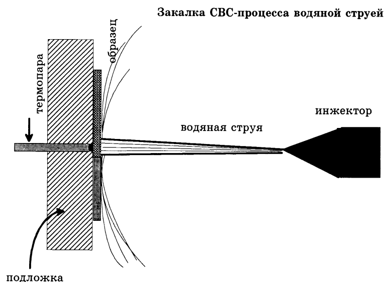
Рис. 24 Схема закалки волны СВС струей воды
