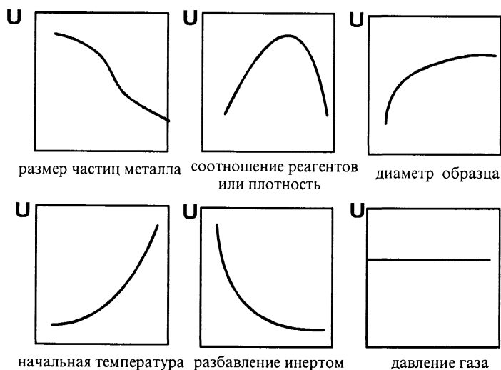
Рис. 20. Схематические зависимости скорости горения от экспериментальных параметров
