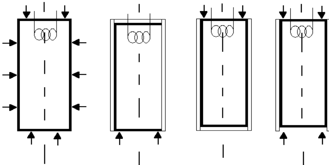
Рисунок 13. Схемы фильтрации газа в системе твердое-газ
