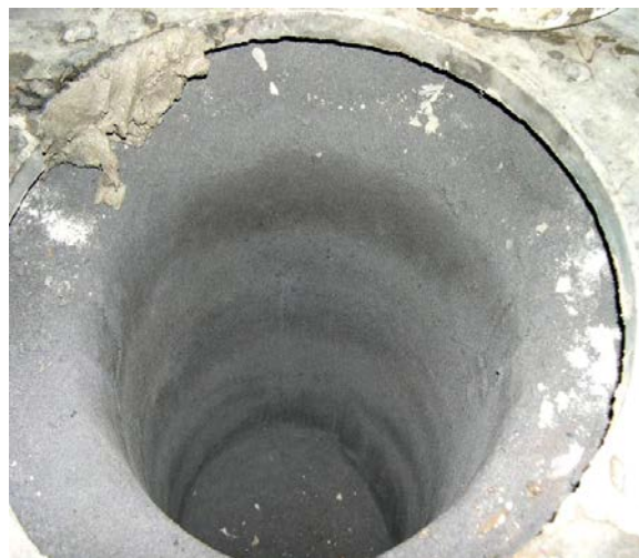
Рис.56 – Футеровка индукционной печи ИСТ-016
