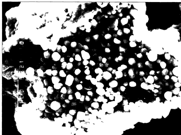
Рис. 30. Микроструктура первичных зерен карбида титана
