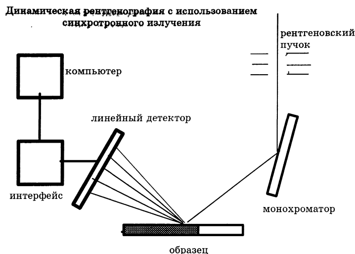
Рис. 22. Схема установки для динамической рентгенографии
