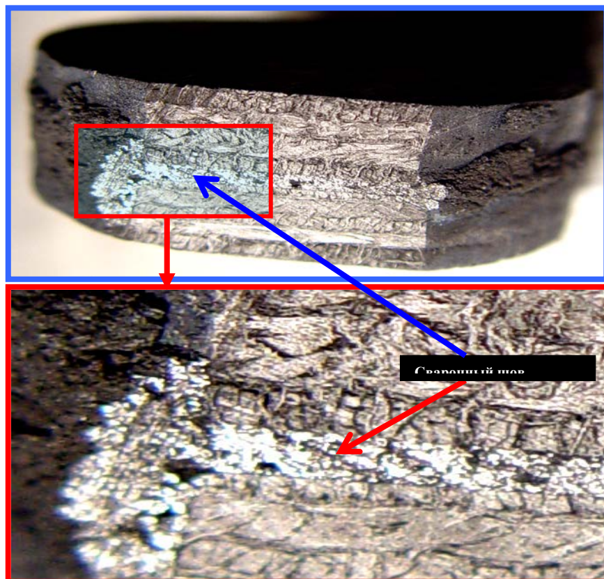
Рис 40 Поперечное сечение СВС-сварки
