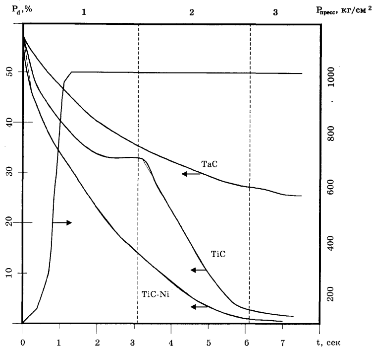
Рис. 39. Механизм уплотнения продуктов горения в процессе СВС-компактирования: 1 — зона скольжения зерен; 2 — область пластической деформации зерен; 3 — область диффузионного залечивания пор.
