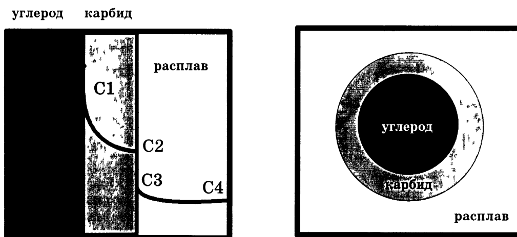
Рис. 7. Схема реакционной ячейки
