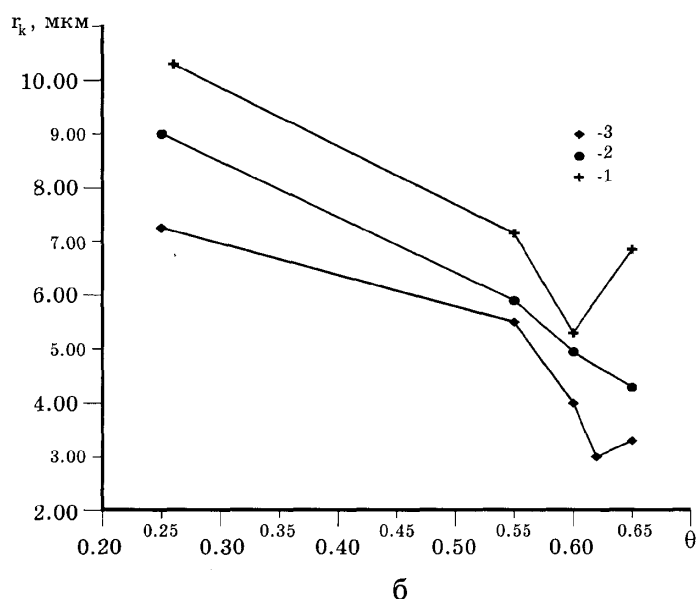
Рис. 47. Зависимости среднего размера зерна карбидной фазы в сплавах, полученных СВС-компактированием, от дисперсности порошка титана в смеси Ti+C (а) и от плотности \theta шихтового брикета (б):
