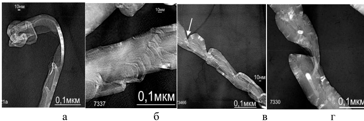
Рисунок 60 – Электронно-микроскопические снимки поверхностей наночастиц
