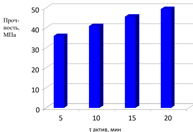
Рисунок 62 – Зависимость прочности на сжатие образцов после СВ-синтеза зауглероженного диоксида кремния от времени активации
