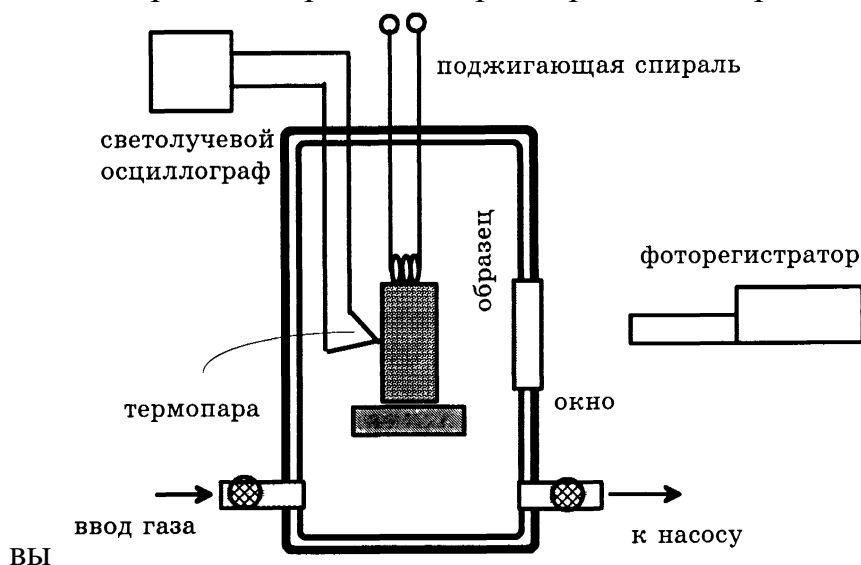
Рис. 19. Схема реакционной камеры для лабораторного исследования СВС-процессов
