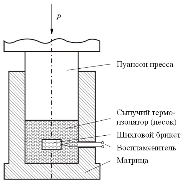
Рисунок 36 -. Схема процесса СВС–прессования
