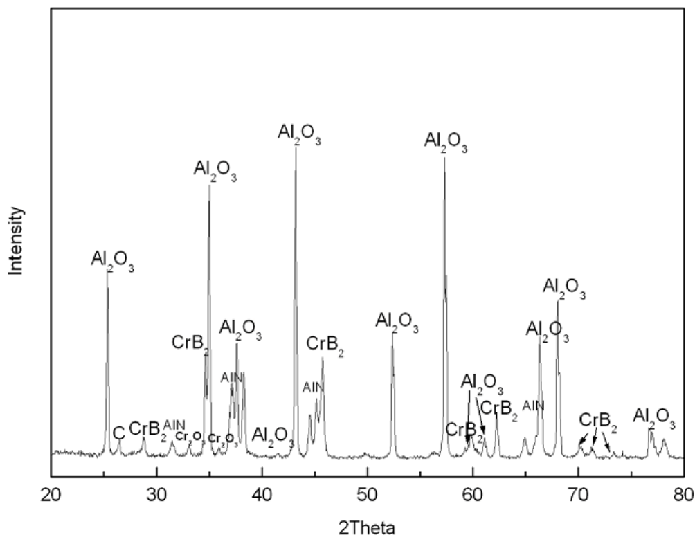
Рисунок бб – Рентгенофазовый анализ СВС-продукта для системы \text{Cr}_2\text{O}_3\text{-B}_2\text{O}_3\text{-Al}
