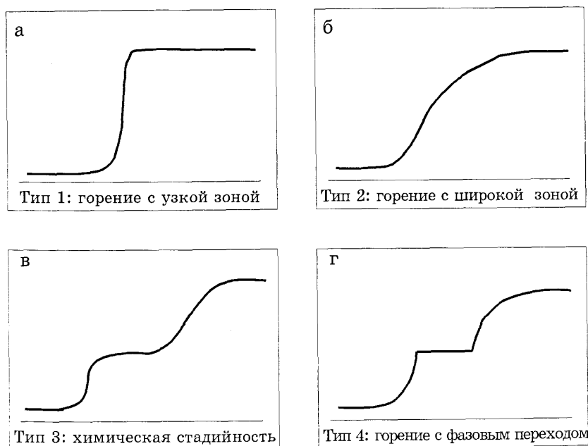
Рис. 1. Типы температурных профилей при СВС
