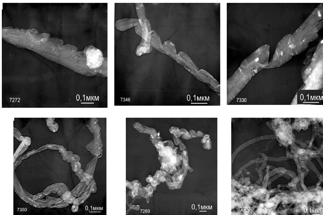
Рисунок 59 – Электронно-микроскопические снимки углеродных наночастиц, полученных зауглероживанием кварца после МА
