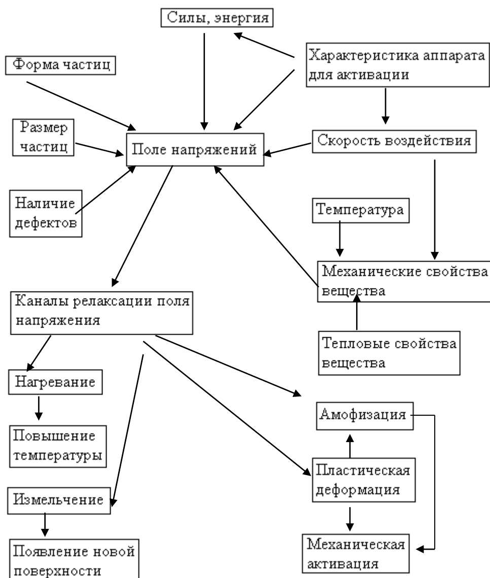
Рисунок 52 – Факторы, влияющие на формирование поля напряжений, и основные каналы релаксации напряжений
