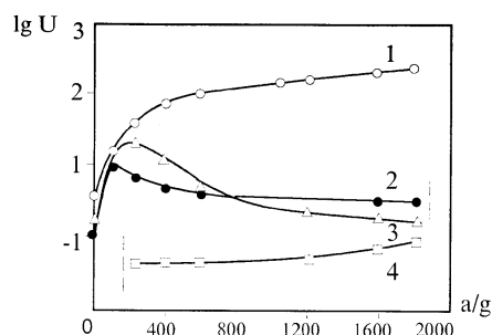
Рис. 46. Влияние перегрузки на скорость горения. Исходные смеси:
