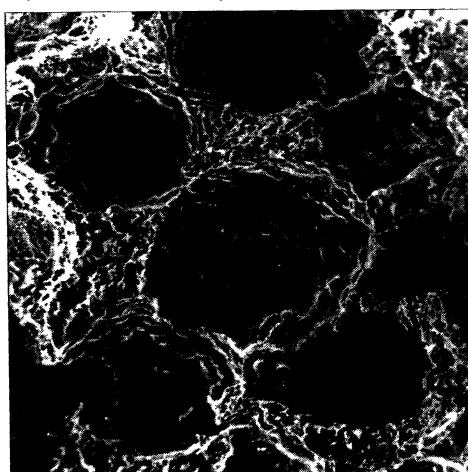
Рис.6б. Капиллярное растекание (впитывание) в системе Ti-C: зона реакции
