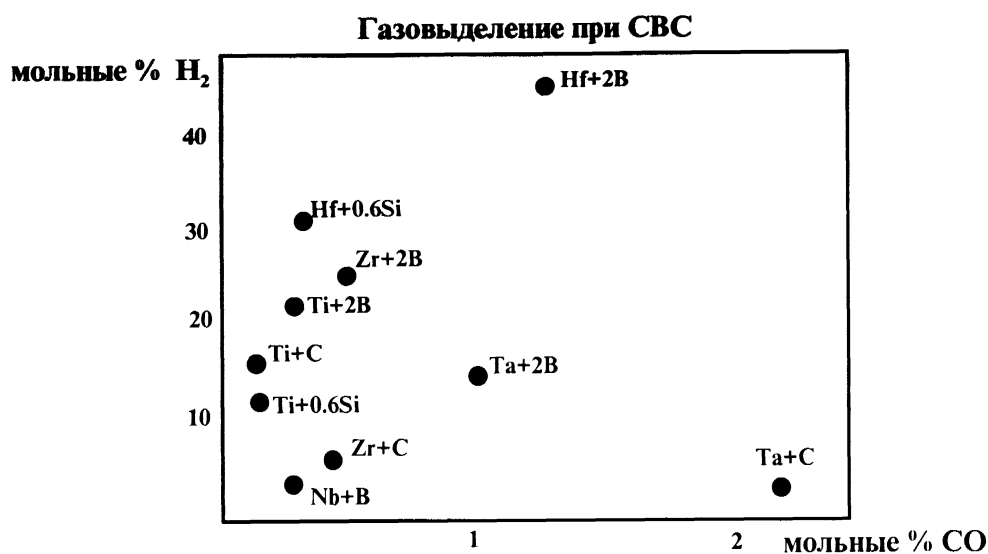
Рис. 12. Относительное содержание водорода и угарного газа в газообразных продуктах, образующихся при СВС
