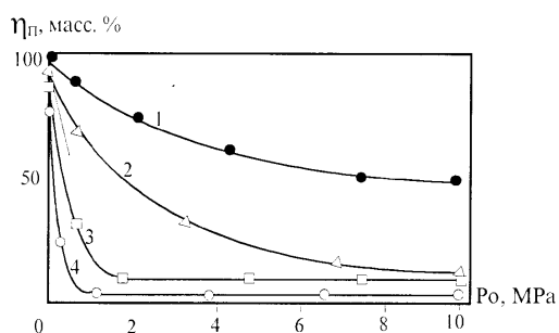
Рис. 42. Влияние начального давления аргона ( P_0 ) на величину потери вещества при горении ( \eta_{\text{п}} ). Исходные смеси:
