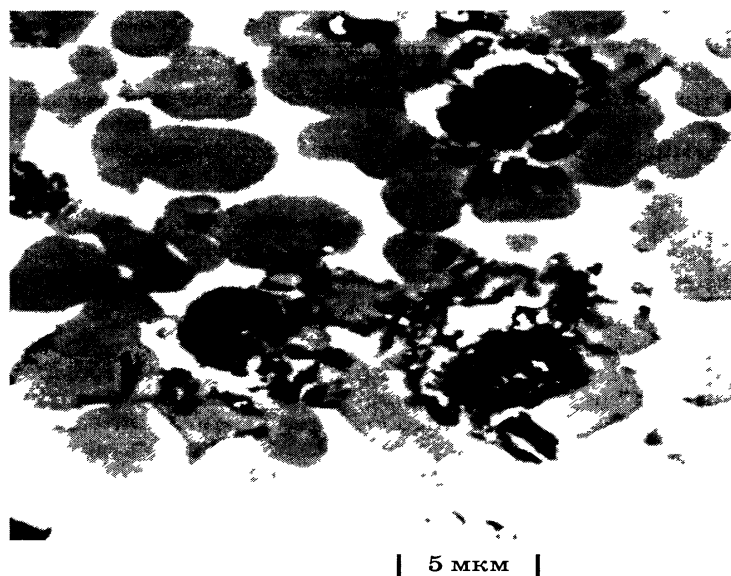
Рис. 8. Взаимодействие углеродных нитей с титановым расплавом
