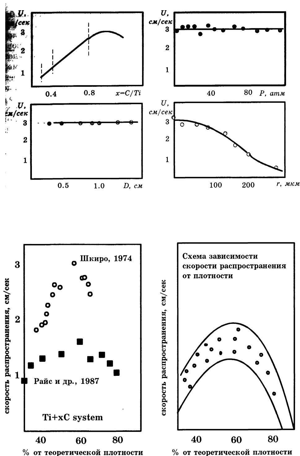
Рис. 4. Зависимости скорости горения в системе Ti+xC от соотношения реагентов ( x ), давления газа ( P ), диаметра образца ( D ), размера частиц титана ( r ) и относительной плотности
