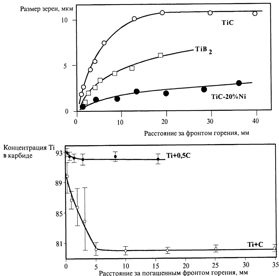
Рис. 31. Зависимость размеров и состава зерен продукта от расстояния за фронтом горения
