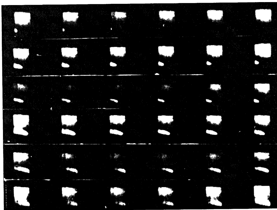
Рис. 15. Кинокадры спинового горения гафния в азоте
