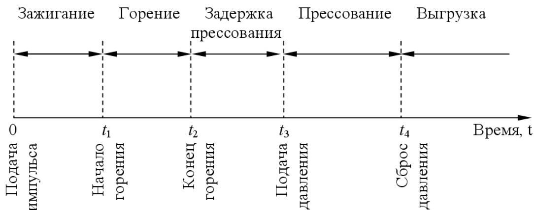
Рисунок 37. Временная диаграмма процесса СВС–прессования
