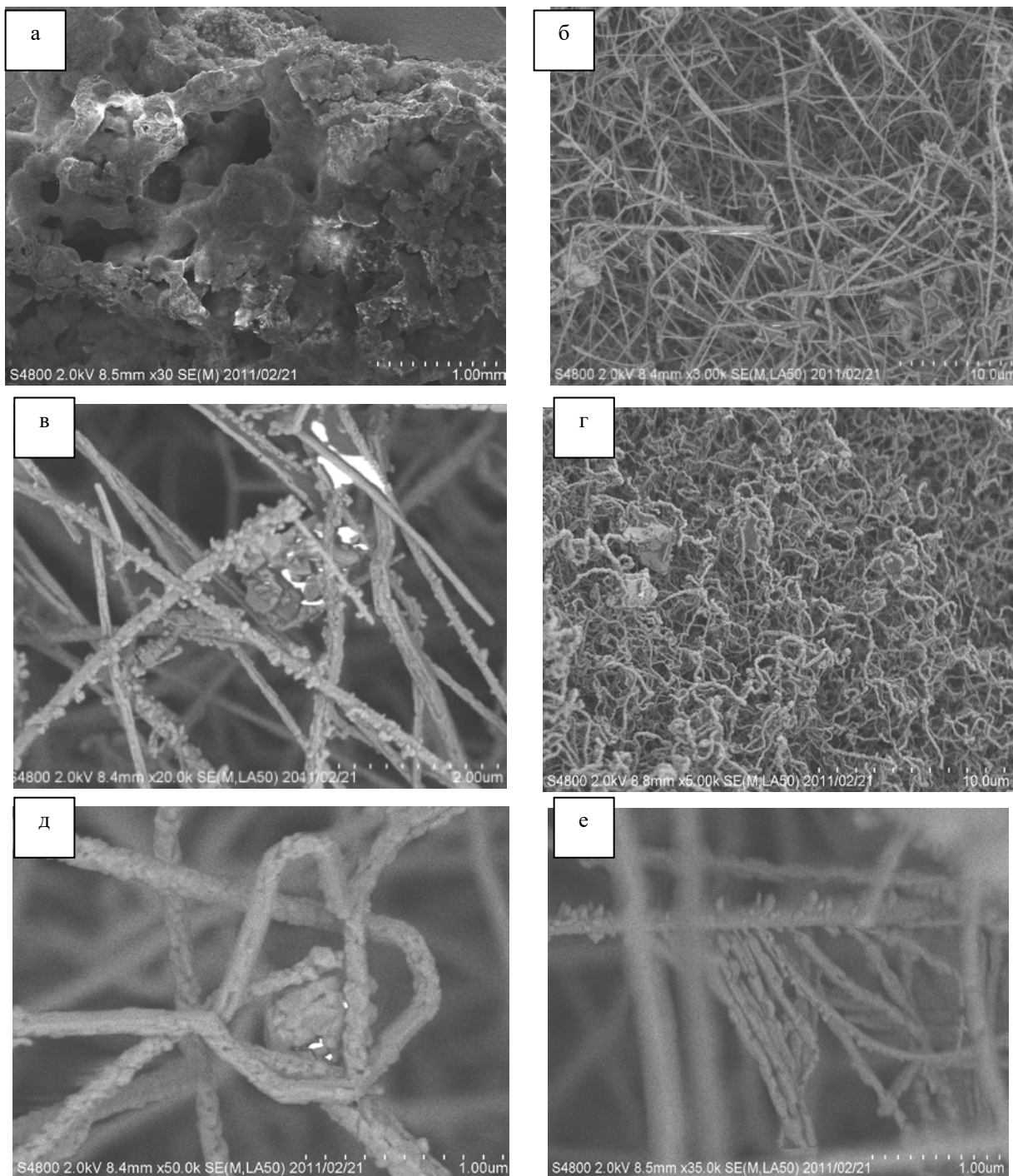
(а) общий снимок поверхности конечных продуктов, (б) нитевидные кристаллы (усы) из оксида алюминия, в, г, д – прямая, волнистая и скрученная формы нитевидных кристаллов, е-разветвление нескольких кристаллов
