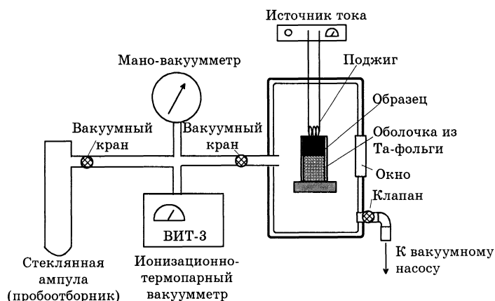
Рис. 27. Схема установки для исследования примесного газовыделения при СВС
