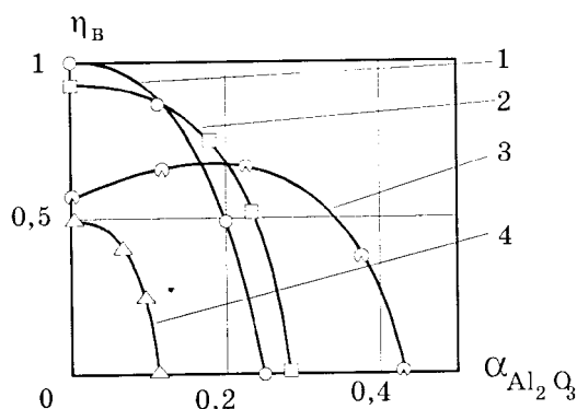
Рис. 44. Влияние массовой доли оксида алюминия в исходной смеси ( \alpha_{Al_2O_3} ) на полноту выхода металлической фазы в слиток ( \eta_B ). Исходные смеси: 1— WO_3 : CoO : Al : C , 2— MoO_3 : Al : C , 3— CrO_3 : Al : C , 4— V_2O_5 : Al : B_2O_3
