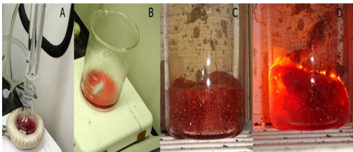
Рис 67 Me^n(NO_3)_n + (n \cdot f) CH_2NH_2CO_2H + n \cdot (f-1) O_2 \Rightarrow MeO_{n/2}(s) + (n \cdot f) CO_2(g) + f H_2O(g) + n \cdot (f+1)/2 N_2(g)
