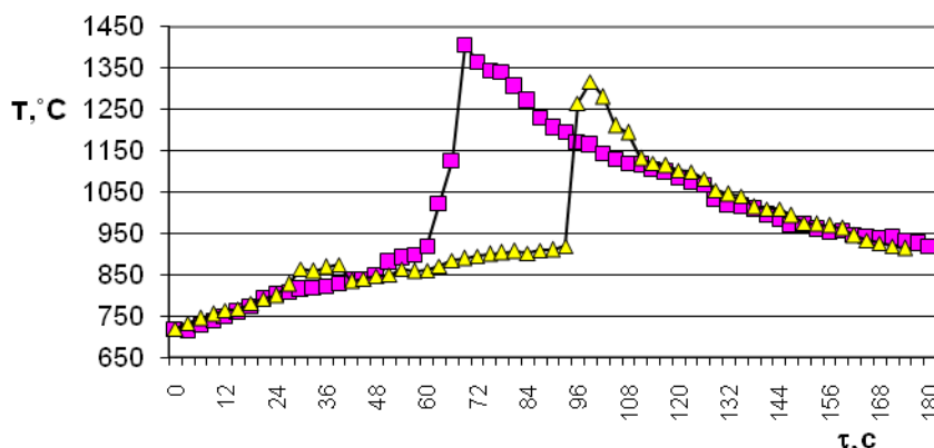
Рисунок 61 – Термограмма процесса горения для зауглероженных систем \text{SiO}_2 -Al
