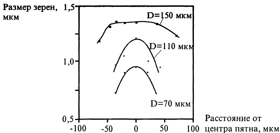
Рис. 34 Распределение размеров зерен NbB_2 по диаметру пятна продукта
