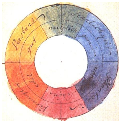
1-сурет. Гетенің түстік шеңбері
