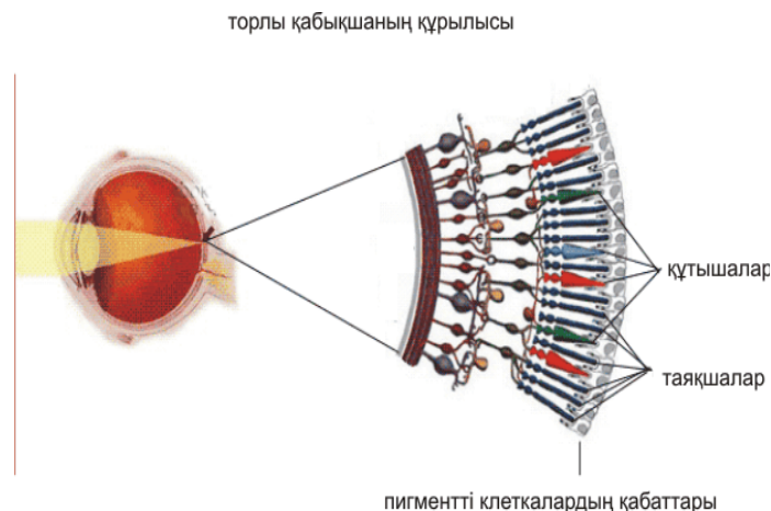
4-сурет. Көз құрылысында құтышалар мен таяқшалардың орналасуы
