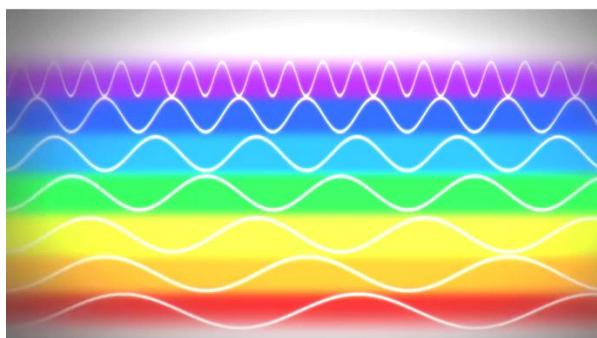
5-сурет. Қызыл түстен көк түске дейінгі түстік спектрдің белгілі бір қатынастағы электромагниттік толқындар
