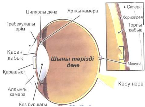
2-сурет. Көздің құрылысы
