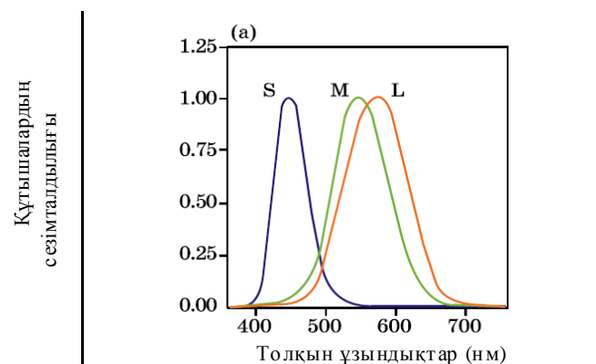
3-сурет. Толқын ұзындықтары
