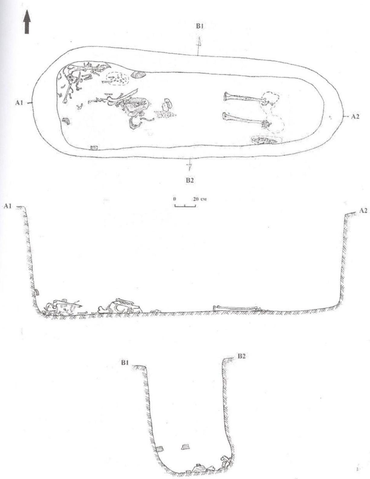
Рис. 4. Могильник Сункар, курган 2. План и разрезы могильной ямы
