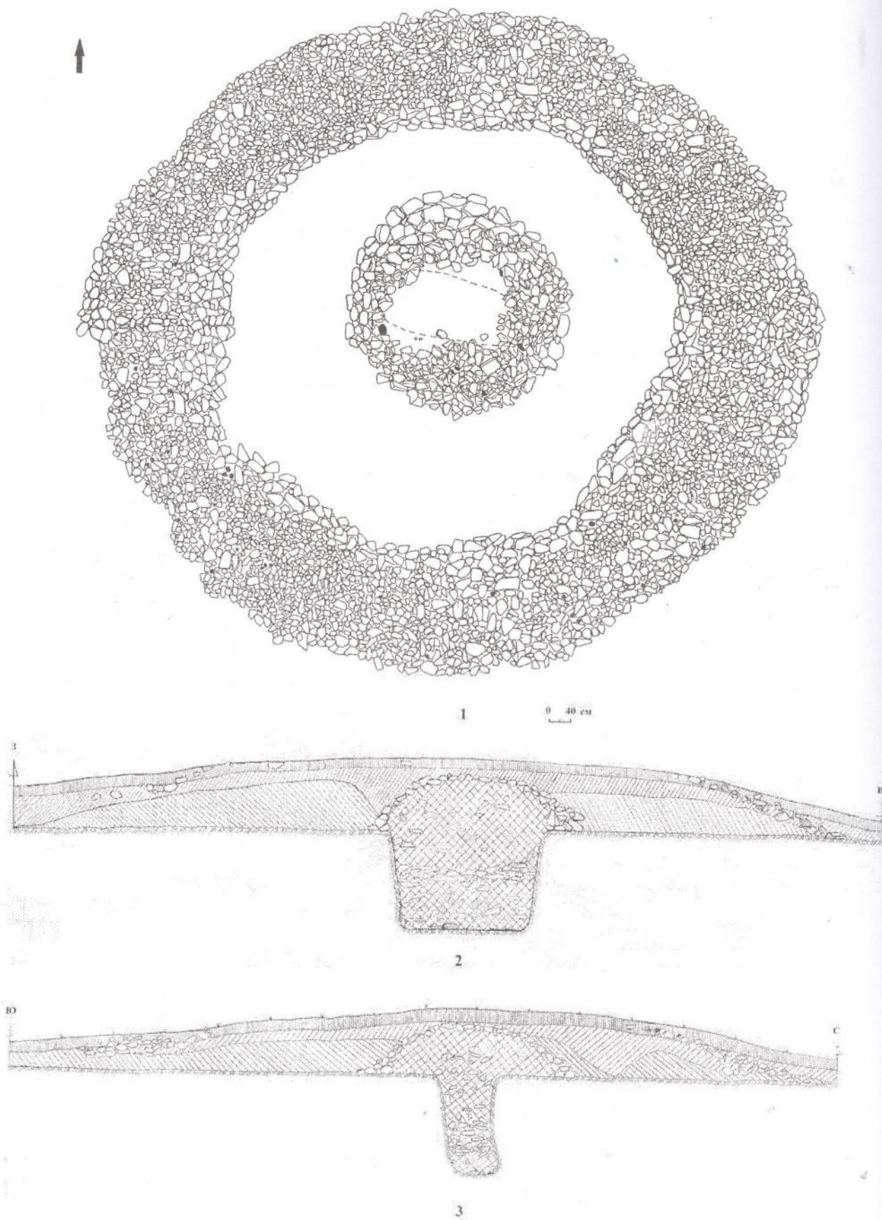
Рис. 3. Могильник Сункар, курган 2. Общий план и разрезы насыпи.
