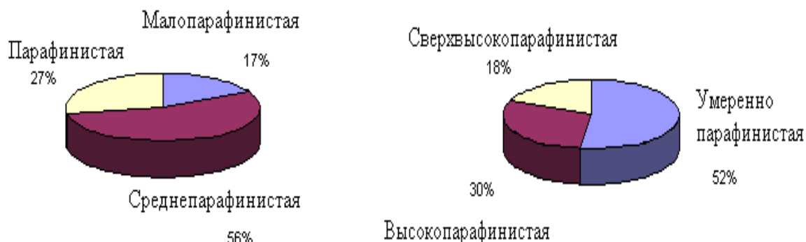
Рисунок 1. Распределение нефтей мира по содержанию парафинов согласно классификации, представленной в табл. 2
