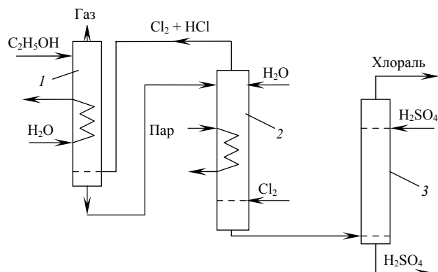
Рис. 15. Реакционный узел для получения хлорала:
