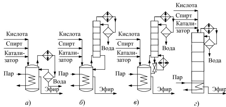
Рис. 36. Реакционные узлы для жидкофазных процессов этерификации, совмещенных с отгонкой азеотропной смеси: а – куб с конденсатором; б – куб с дефлегмирующей колонной; в – куб с ректификационной колонной; г – реактор типа тарельчатой колонны
