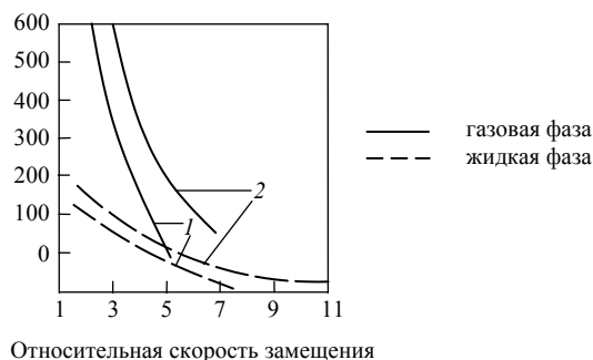
Рис. 2. Температурная зависимость относительной скорости замещения различных атомов водорода при хлорировании парафинов:
