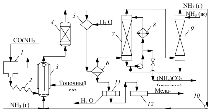
Рис. 39. Технологическая схема производства меламина из карбамида:
