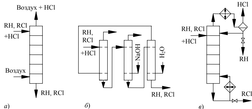
Рис. 7. Схемы очистки продуктов хлорирования от HCl:
