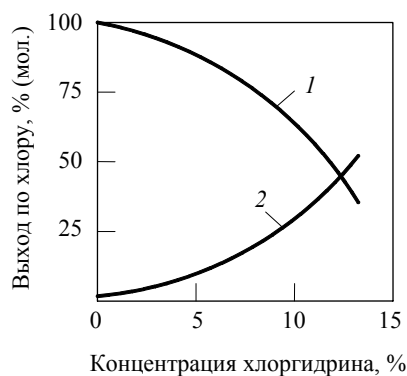
Рис. 12. Зависимость выхода хлоргидрина (1) и дихлорида (2) при хлоргидринировании этилена от концентрации хлоргидрина в растворе
