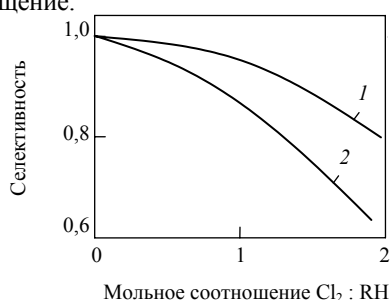
Рис. 4. Зависимость селективности от мольного отношения превращенного хлора к парафину или хлорпарафину: 1 – первый продукт замещения; 2 – второй продукт замещения при возвращении промежуточного вещества на реакцию
