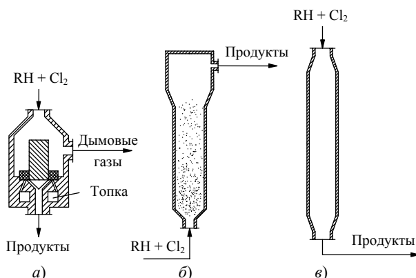
Рис. 9. Реакторы для газовой фазы хлорирования с насадкой-теплоносителем (а), с псевдоожиженным слоем теплоносителя (катализатора) (б) и с предварительным подогревом смеси (в)
