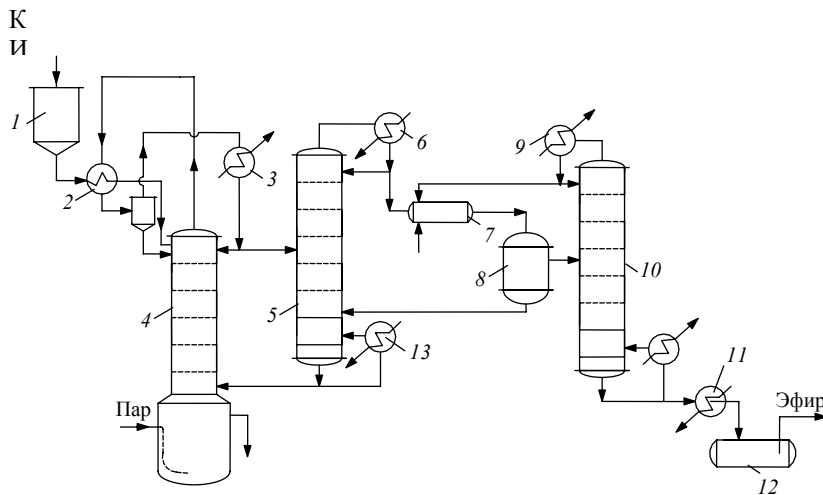
Рис. 37. Технологическая схема непрерывного производства этилацетата: 1 – напорный бак; 2 – теплообменник; 3 – конденсатор; 4 – эфиризатор; 5, 10 – ректификационные колонны; 6, 9 – конденсаторы-дефлегматоры; 7 – смеситель; 8 – сепаратор; 11 – холодильник; 12 – сборник; 13 – кипятильник
