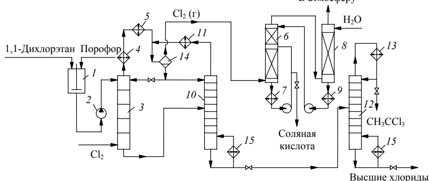
Рис. 8. Технологическая схема получения 1,1,1-трихлорэтана:
