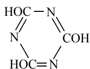
циануровая кислота
