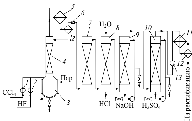
Рис. 24. Технологическая схема производства фреона-12:
