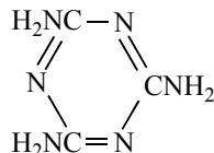
меламин
