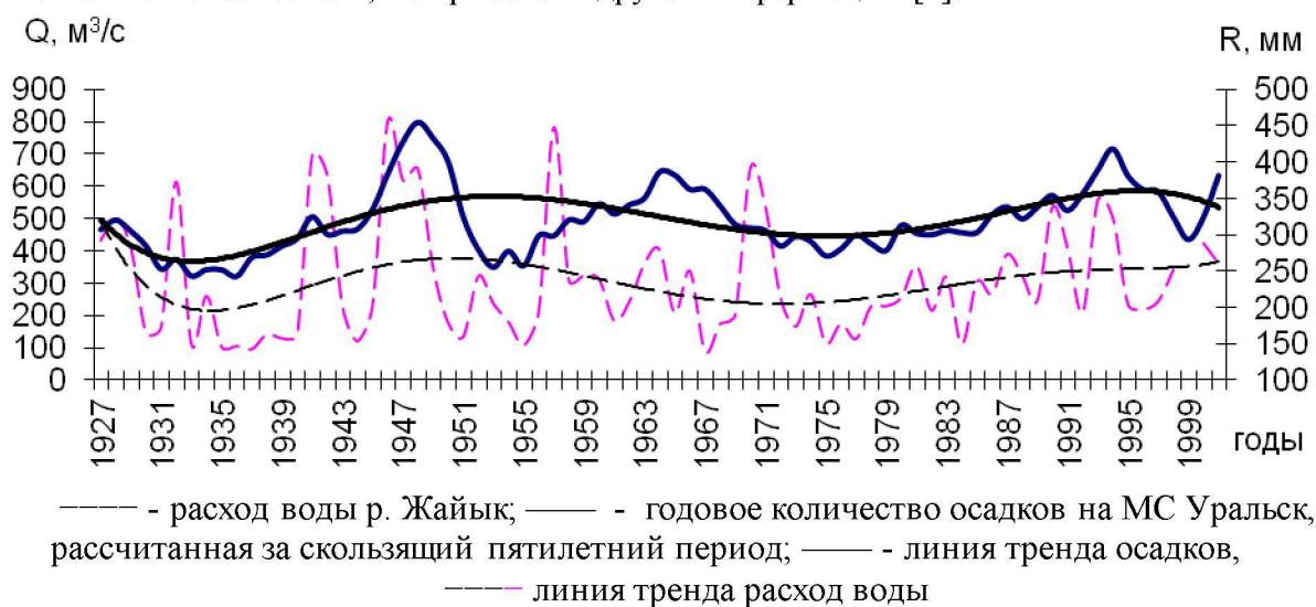
Рисунок 2. Временной ход расхода воды р. Жайык и годовой суммы осадков на МС Уральск, рассчитанные за скользящий пятилетний период
