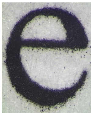
Фото №5. Микроструктура штрихов печатного текста, выполненного на лазерном принтере. (увел. 32х)
