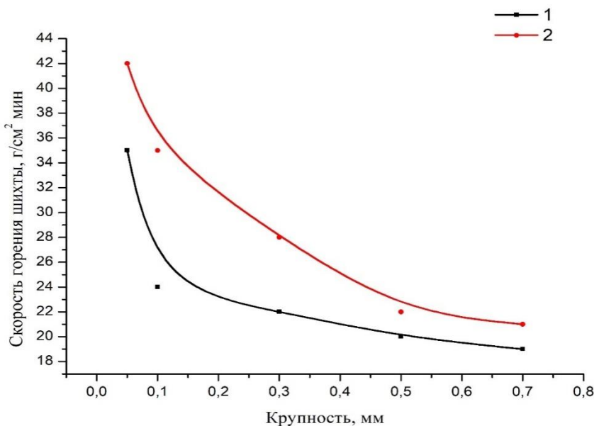
Рисунок 1 – Зависимость скорости проплавления шихты от крупности алюминия при стехиометрическом соотношении компонентов
