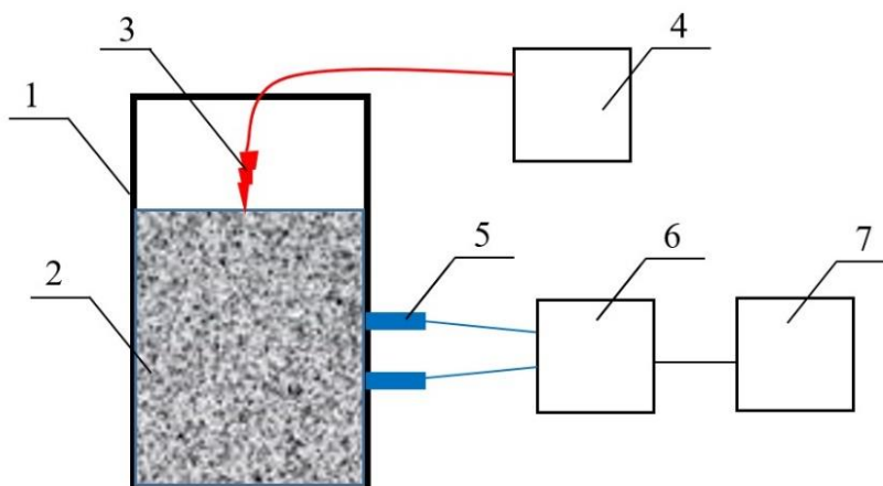
Рисунок 2 – Схема установки для определения скорости горения шихты
