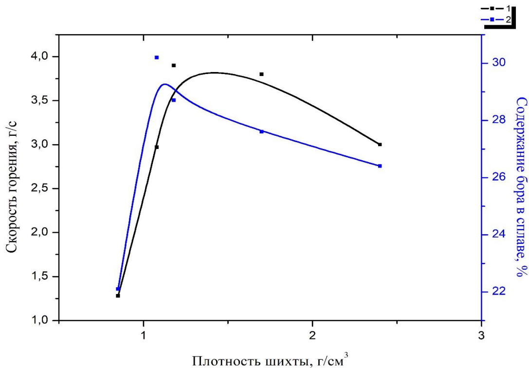
Рисунок 3 – Влияние плотности шихты на скорость горения и содержание бора в сплаве
