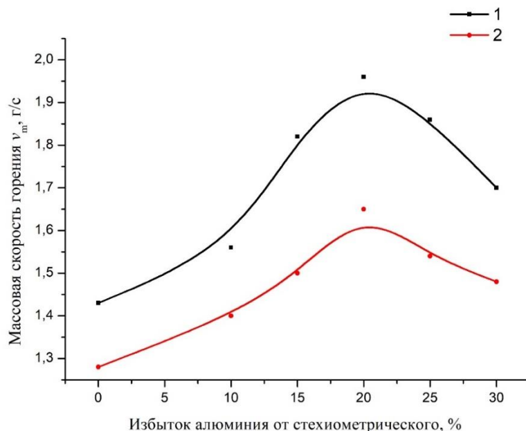
Рисунок 4 – Зависимость скорости горения шихты от дисперсности и избытка алюминия 1 – крупность алюминия 0,10-0,25 мм; 2 – крупность алюминия 0,40-0,50 мм
