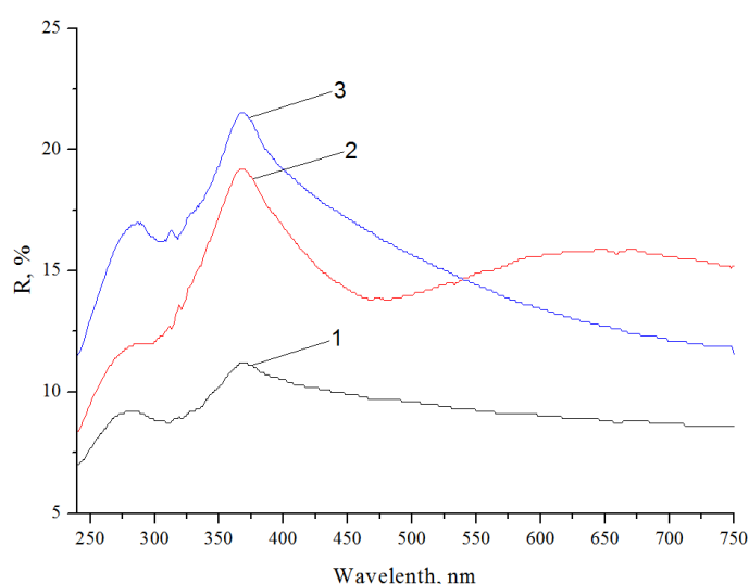
1 - J = 1\text{ мА/см}^2 , t = 20\text{ мин} ; 2 - J = 10\text{ мА/см}^2 , t = 2\text{ мин} ; 3 - J = 20\text{ мА/см}^2 , t = 1\text{ мин}
