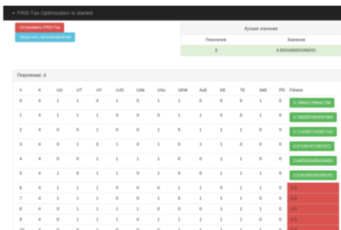
Рис. 11. Результаты выполнения генетического алгоритма, поколение 3
