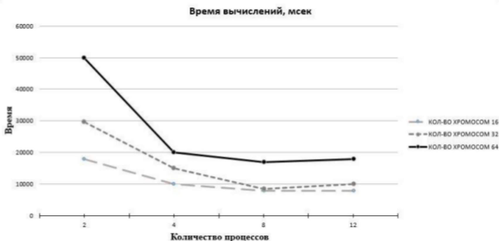
Рис. 7. Время вычислений параллельного алгоритма FRiS-Tax
