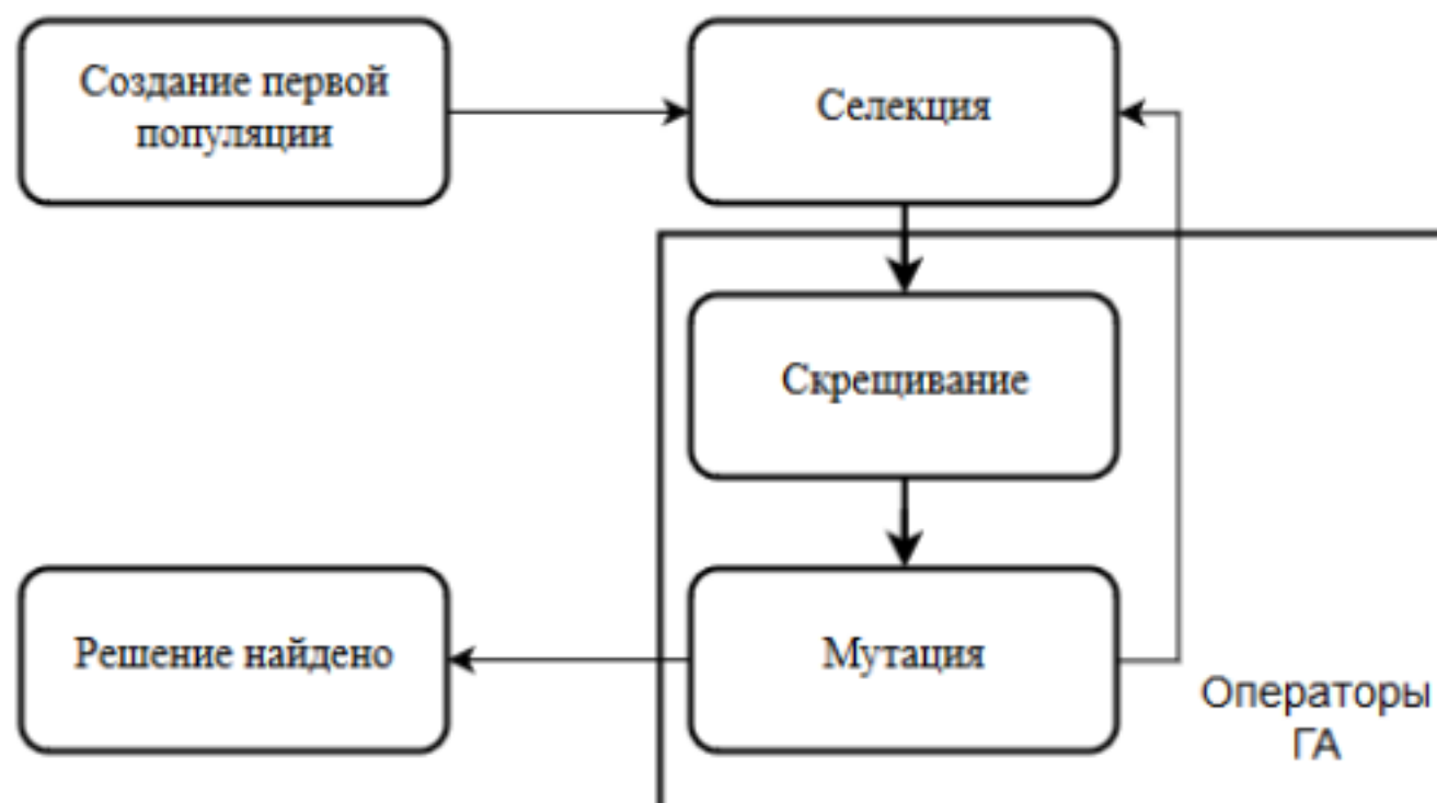
Рис. 2. Схема генетического алгоритма
