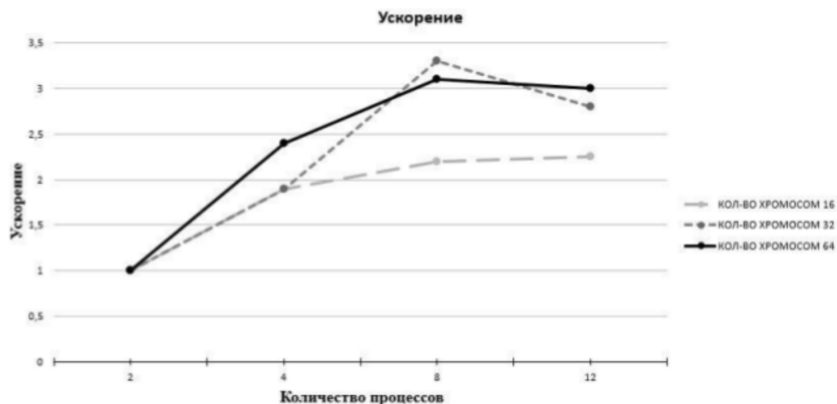
Рис. 8. Ускорение параллельного алгоритма FRiS-Tax
