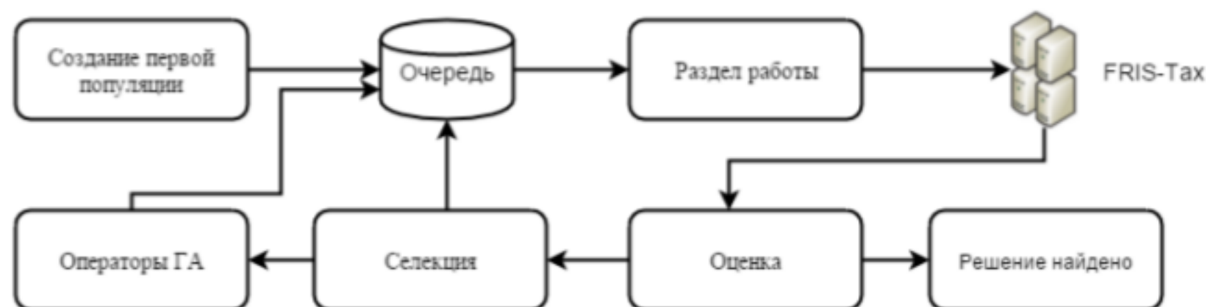
Рис. 6. Схема параллельного алгоритма кластеризации FRiS-Tax
