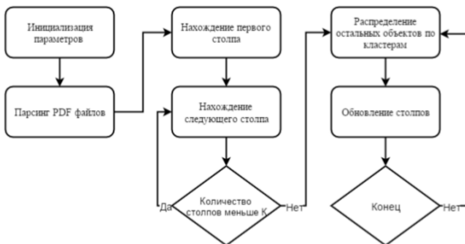
Рис. 1. Алгоритм кластеризации FRiS-Tax
