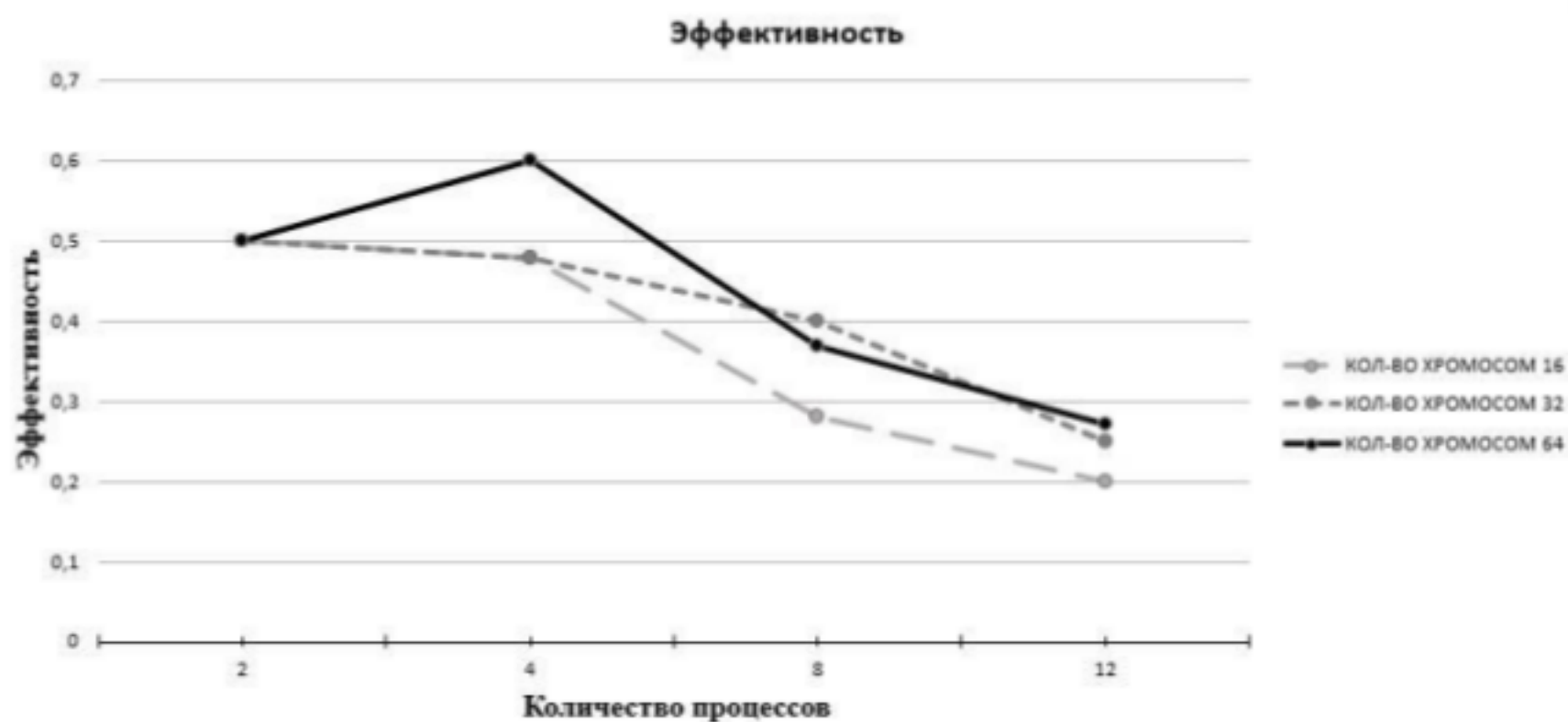
Рис. 9. Эффективность параллельного алгоритма FRiS-Tax
