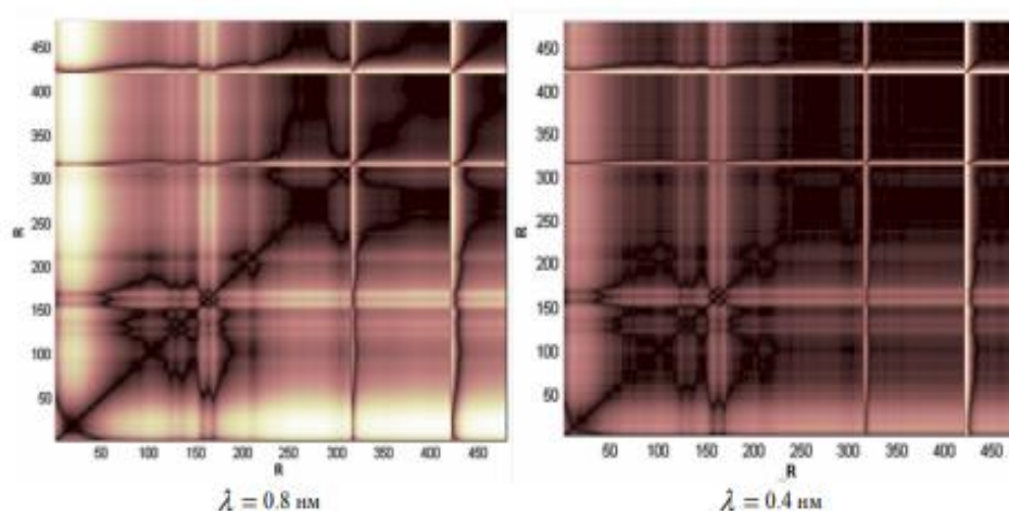
2-сурет – Әр түрлі толқын ұзындығы мәніндегі рентгендік сәуле шығарудың рекуренттік диаграммасы 23.10.2012 ж., \varepsilon = 0,2 , \rho = 0,5
