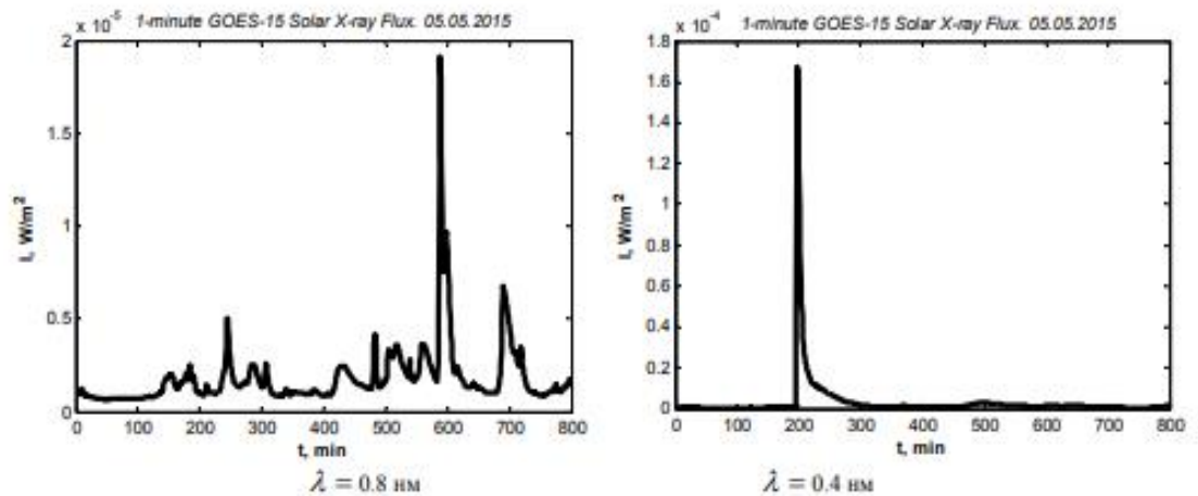
1-сурет – Рентгендік сәуле шығару (5/05/2015)
