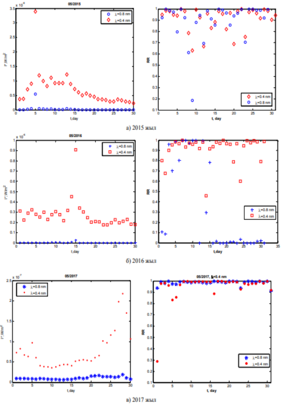
3-сурет – Мамыр айы үшін әр түрлі жылдағы әр түрлі толқын ұзындығындағы рентгендік сәуле шығарудың орташа мәні (сол жақта) және олардың рекурренттілік өлшемі (оң жақта)
