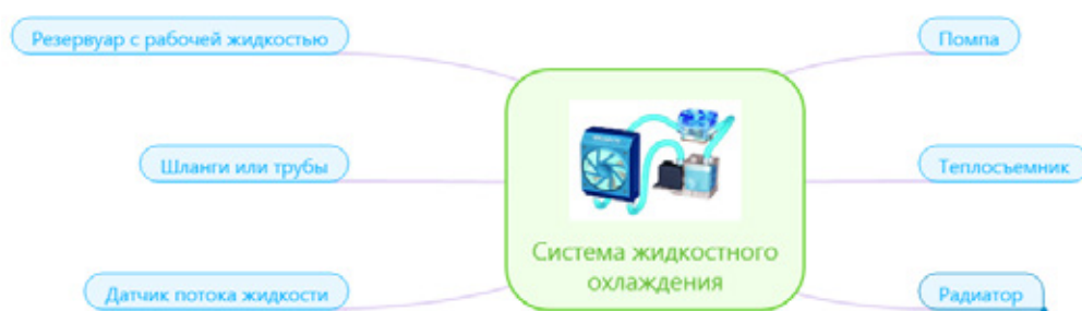
Рис. 2.1. Диаграмма связей системы жидкостного охлаждения
