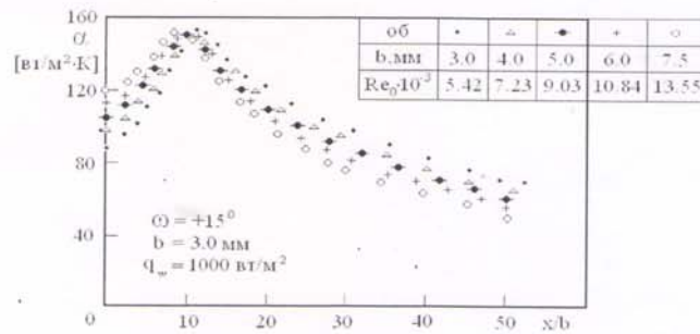
1-сурет – Айырылысатын конустық ағындағы жергілікті жылуалмасу коэффициенті
