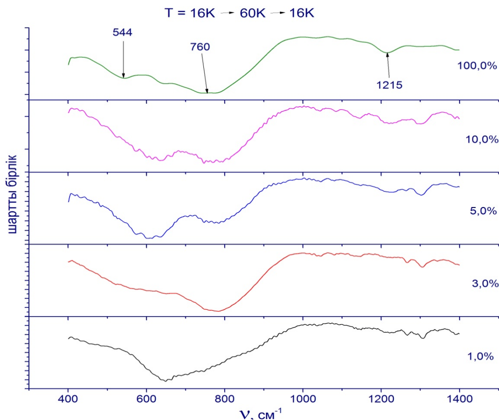
5-сурет – Реконденсаттардың және 100,0%-дық үлгінің ИҚ-спектрлері. 400-1400 \text{cm}^{-1} жиіліктер аралығы
