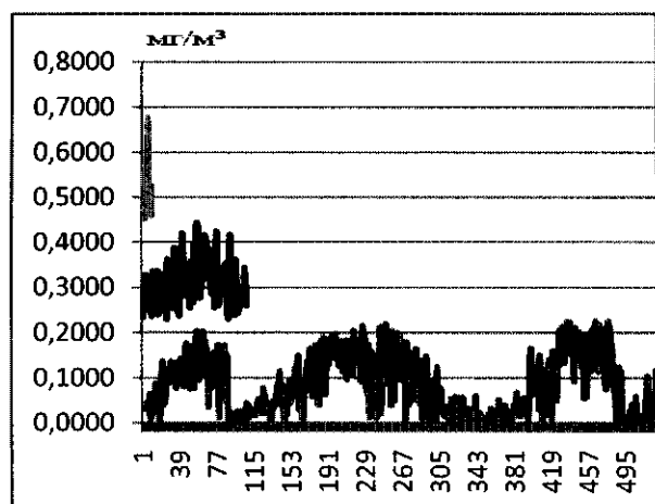
Рисунок 4 – Суточный ход приземного озона за 13 час (2003-2005 гг.)
