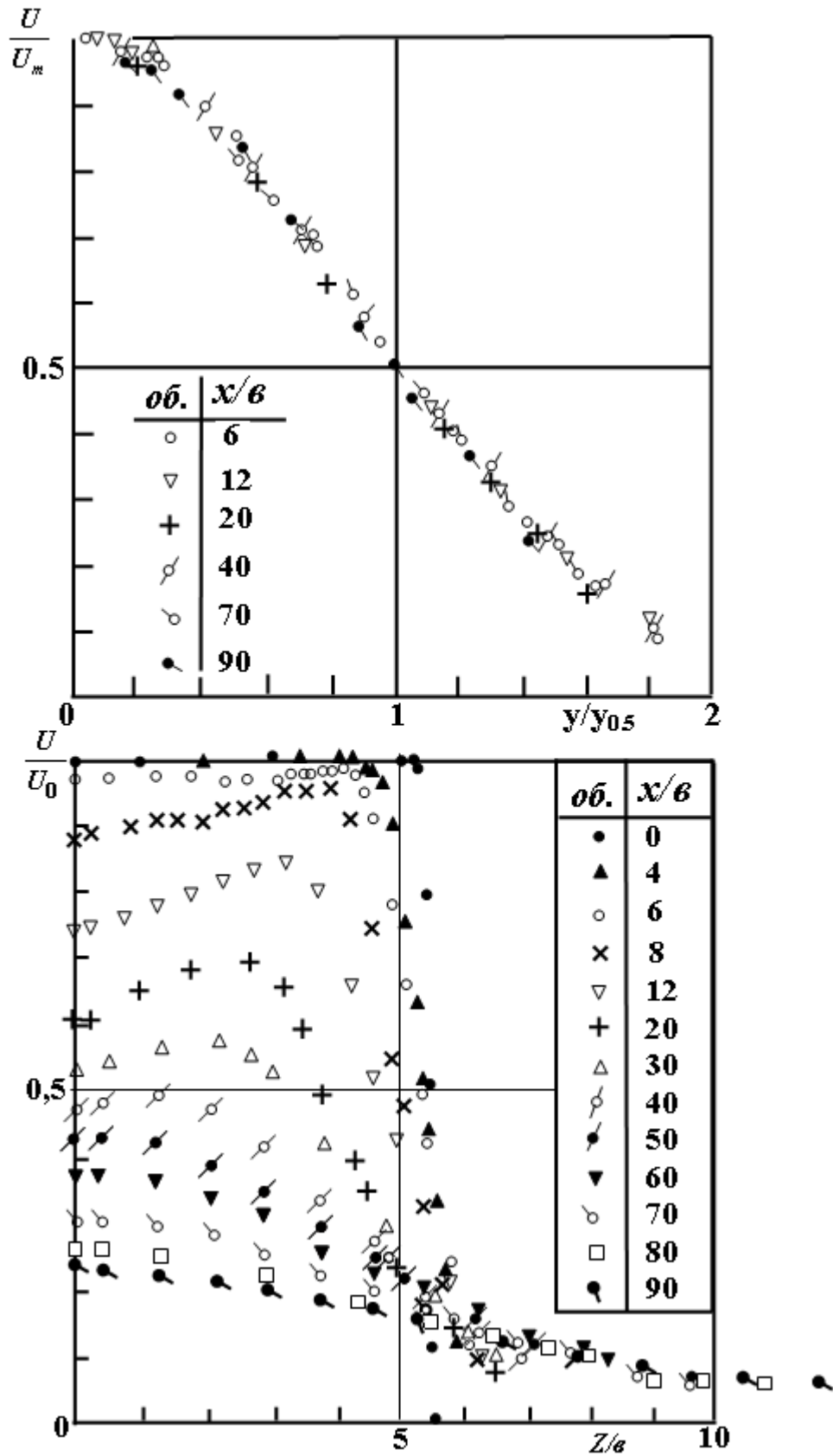
Рис. 3. Безразмерные профили скорости трехмерной струи
