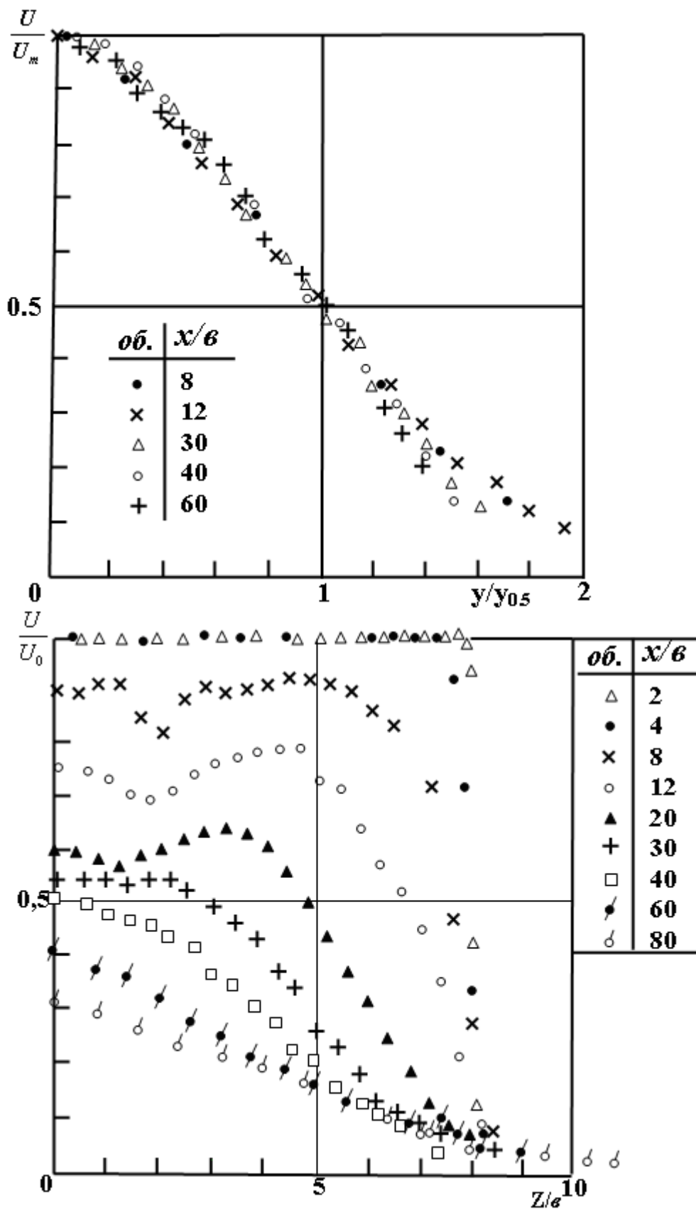
Рис. 4. Безразмерные профили скорости трехмерной струи
