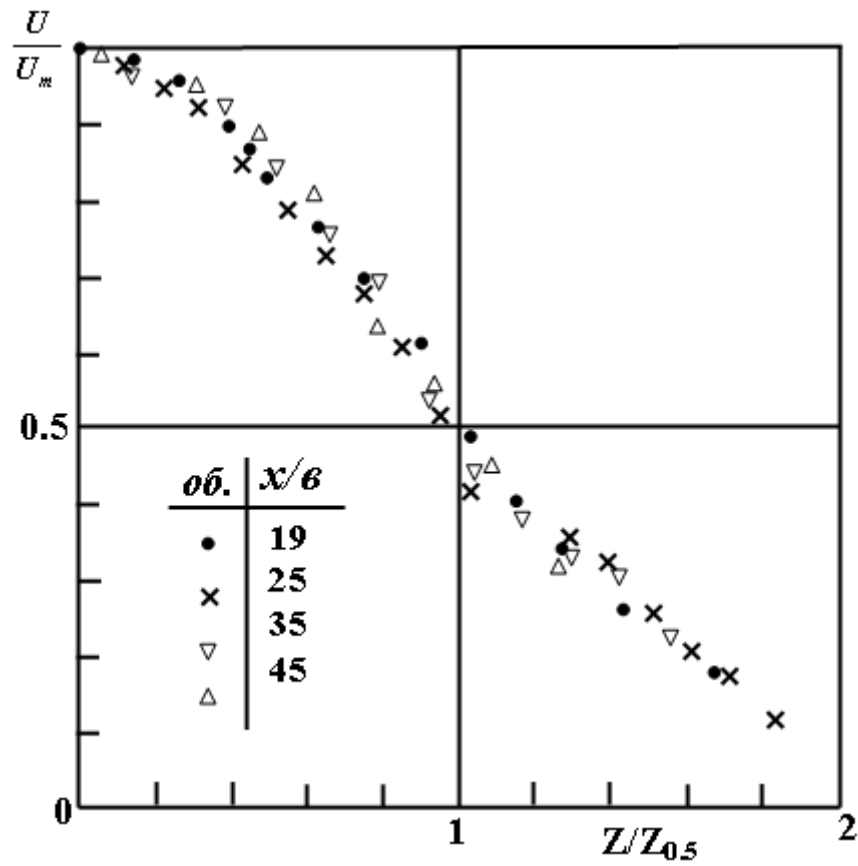
Рис. 2. Безразмерные профили скорости трехмерной струи
