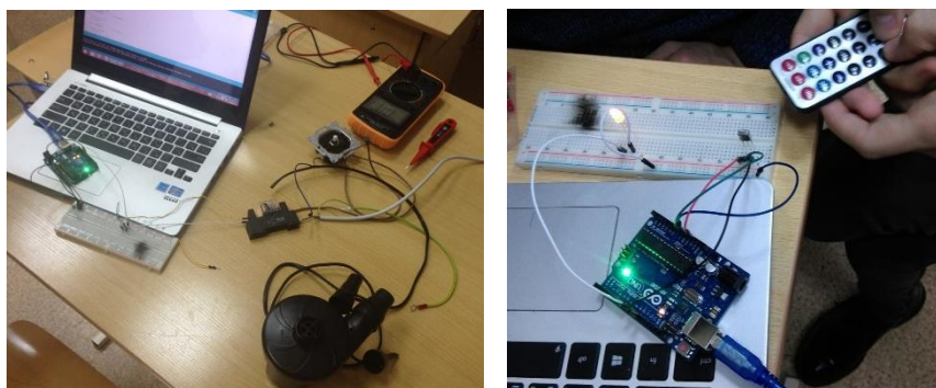
Сурет 5. Аппараттық құрастыру және вентилятор жұмысын пульспен басқару
