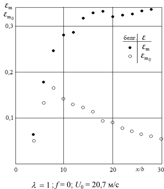
4-сурет. Ағыншадағы турбуленттіліктің интенсивтілігінің осьтік таралуы
