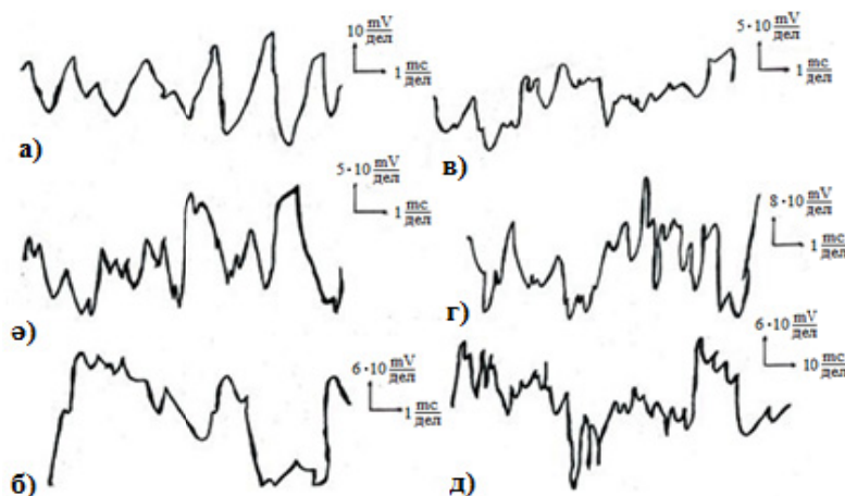
\lambda = 1, U_0 = 20, 7M/c; f = 0; y = 0; z = 0; U_0 — бастапқы жылдамдық; f — сыртқы акустикалық әсер жиілігі; а) x/b=2 ; б) x/b=6 ; в) x/b=10 ; г) x/b=18 ; д) x/b=26 ; е) x/b=30
