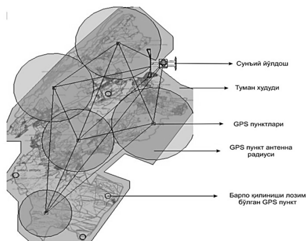
Rasm 2. Suniy yo'ldoshlar orqali joy koordinatalarini aniqlash
