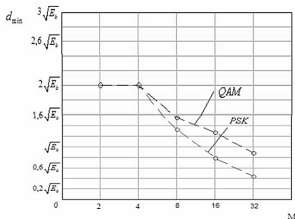
4-rasm. QAM va PSK uchun xalaqitbardoshlikning modulyatsiya holati soni M ga bog'liqligi
