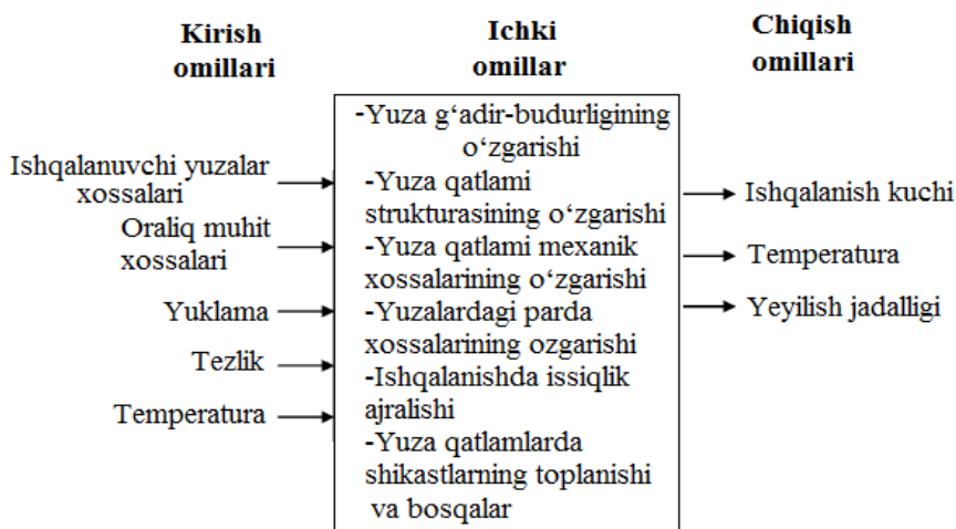
1-rasm. Ishqalanish va yeyilish jarayonini aniqlovchi omillar
