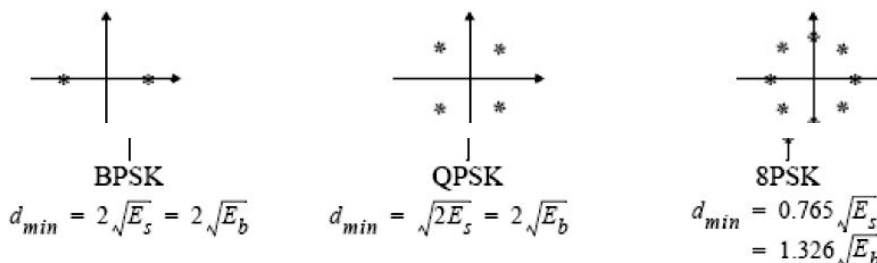
1-rasm. Faza modulyatsiyasi asosiy turlarining signal yulduzchalari
