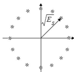
2-rasm. 16PSK faza modulyatsiyali signalning yulduzchalari
