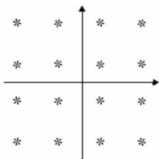
3-rasm. 16QAM modulyatsiyali signalning yulduzchalari
