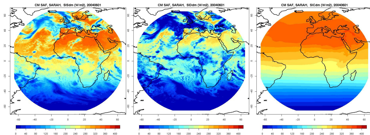
Рисунок 5 – Зона покрытия базы SARAH
