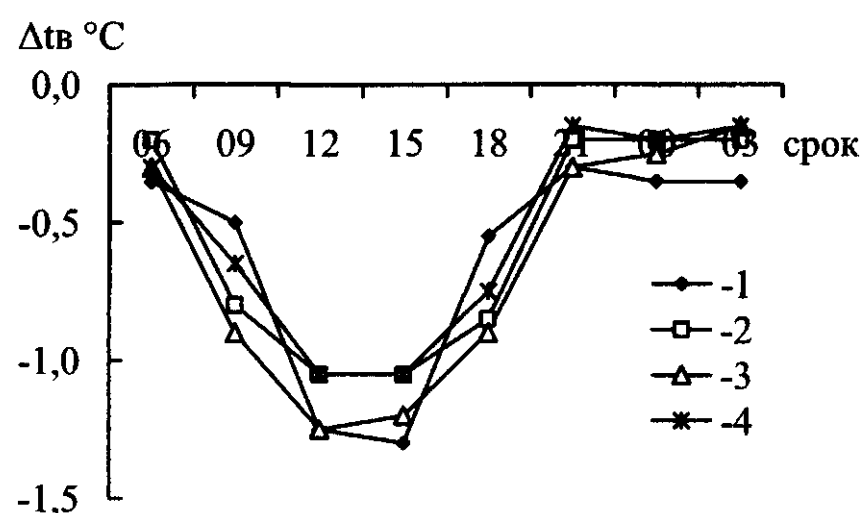
Рис. 1. Суточный ход \Delta t_v по сезонам за 2010 и 2011 годы. 1 – зима, 2 – весна, 3 – лето, 4 – осень.
