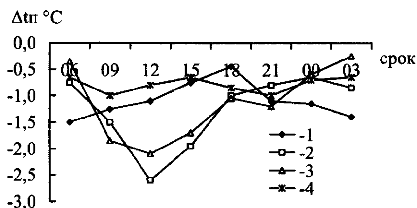
Рис. 2. Суточный ход \Delta t_p по сезонам за 2010 и 2011 годы. 1 – зима, 2 – весна, 3 – лето, 4 – осень.
