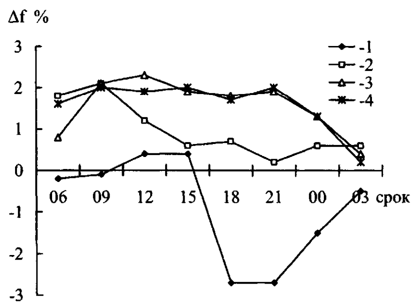
Рис. 4. Суточный ход Δf по сезонам 2010 год. 1 – зима, 2 – весна, 3 – лето, 4 – осень.
